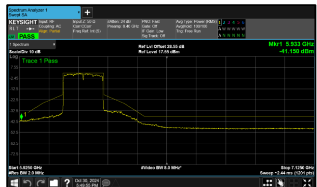
Figure 356 - B (Core 1) 802.11ax HE160 SU SP 6185 MHz (CH47)
