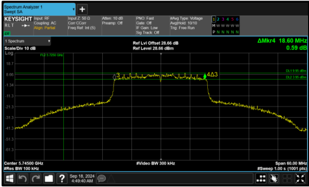
Figure 236 - 802.11ax HE20 SU Minimum 6 dB EBW
