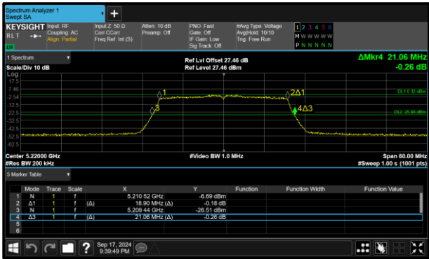
Figure 222 - 802.11ax HE20 SU Minimum 99% OBW
