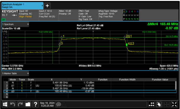
Figure 257 - 802.11ax HE160 SU Maximum 99% OBW
