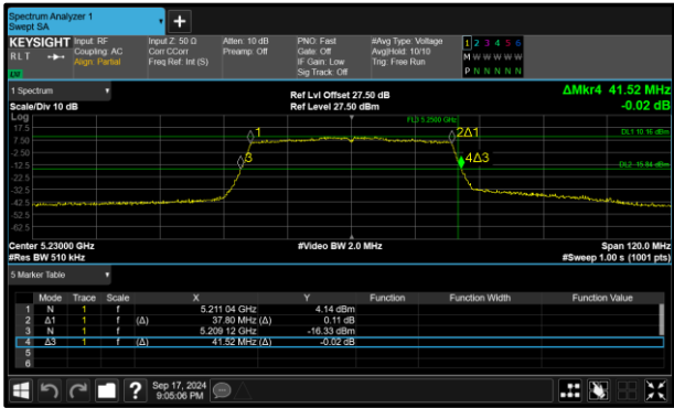
Figure 196 - 802.11ax HE40 SU Minimum 99% OBW
