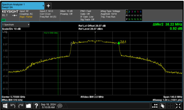
Figure 253 - 802.11ax HE40 SU Maximum 99% OBW
