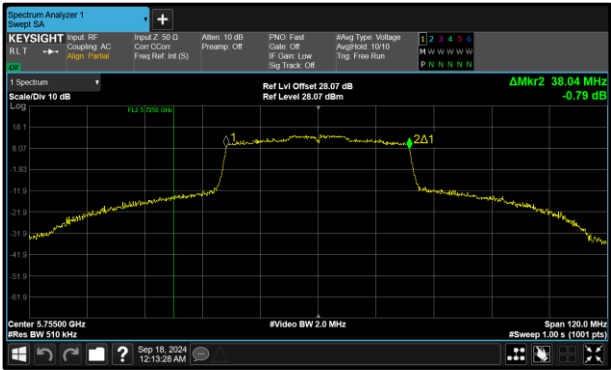
Figure 197 - 802.11ax HE40 SU Maximum 99% OBW
