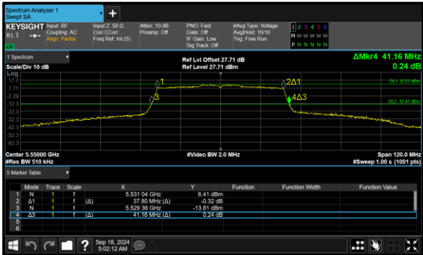
Figure 252 - 802.11ax HE40 SU Minimum 99% OBW
