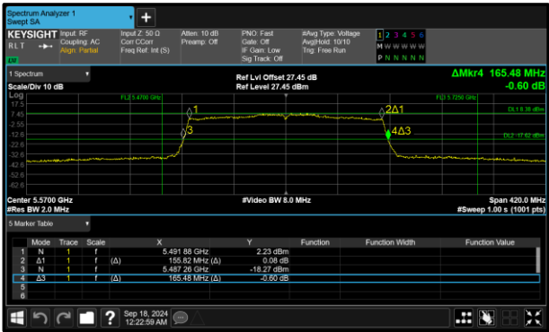
Figure 201 - 802.11ax HE160 SU Maximum 99% OBW
