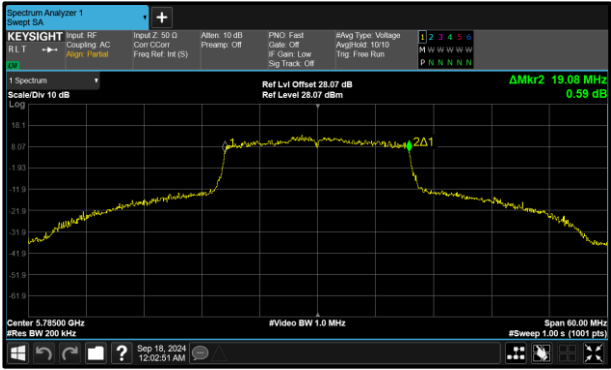
Figure 195 - 802.11ax HE20 SU Maximum 99% OBW
