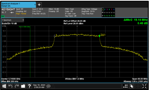
Figure 223 - 802.11ax HE20 SU Maximum 99% OBW
