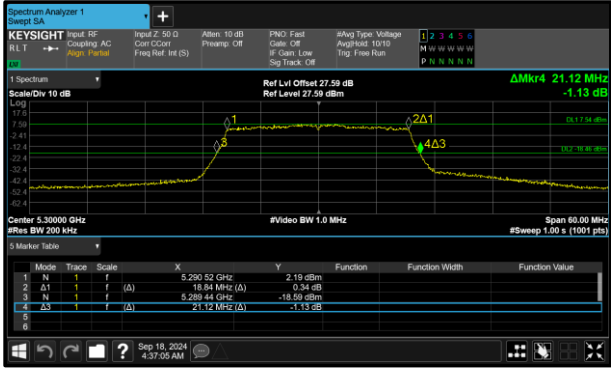
Figure 250 - 802.11ax HE20 SU Minimum 99% OBW
