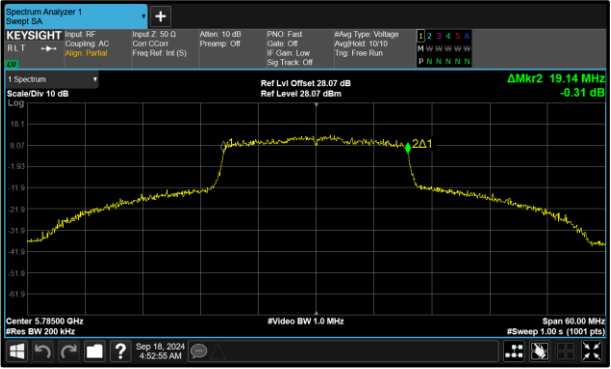
Figure 251 - 802.11ax HE20 SU Maximum 99% OBW
