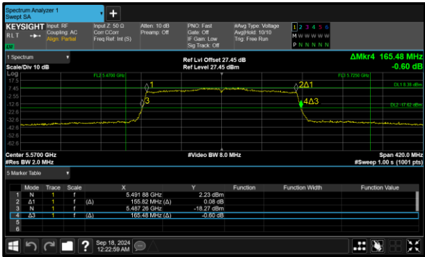
Figure 200 - 802.11ax HE160 SU Minimum 99% OBW
