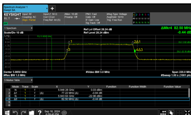
Figure 37 - 802.11ax HE80 SU LPI Minimum 99% OBW
