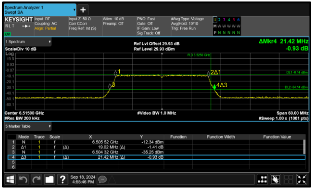
Figure 171 - 802.11ax HE20 SU LPI Minimum 99% OBW
