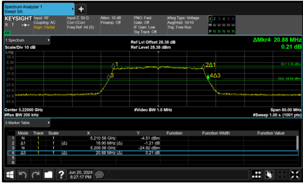
Figure 308 - 802.11ax HE20 SU Minimum 99% OBW
