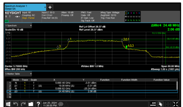
Figure 281 - 802.11ax HE20 SU Maximum 99% OBW
