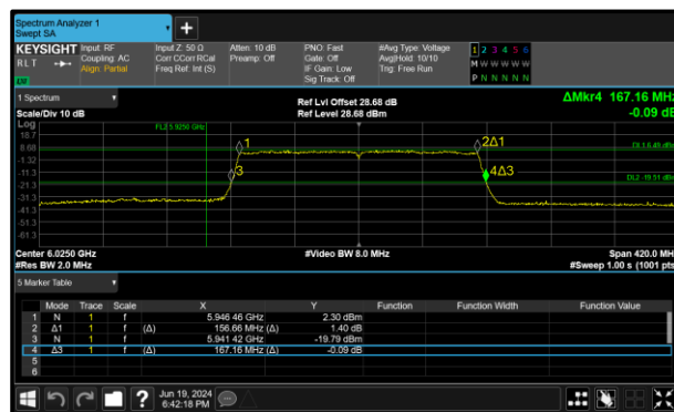
Figure 30 - 802.11ax HE160 SU LPI Maximum 99% OBW
