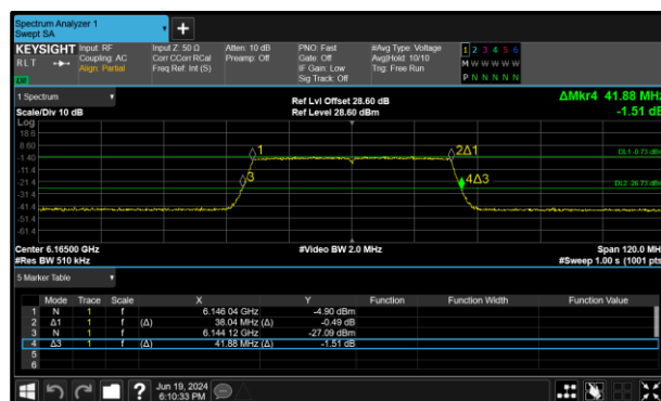
Figure 26 - 802.11ax HE40 SU LPI Maximum 99% OBW
