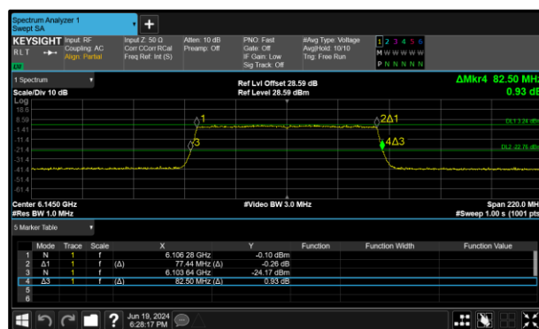
Figure 28 - 802.11ax HE80 SU LPI Maximum 99% OBW
