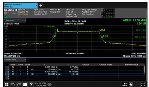
Figure 62 - 802.11ax HE20 SU SP Maximum 99% OBW
