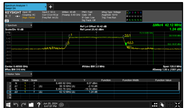
Figure 80 - 802.11ax HE40 SU SP Maximum 99% OBW
