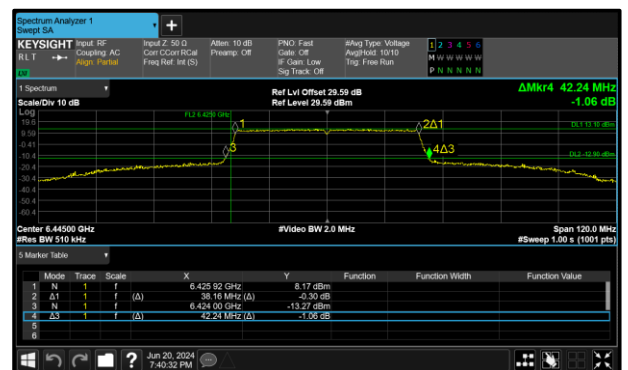
Figure 64 - 802.11ax HE40 SU SP Maximum 99% OBW
