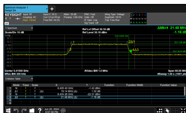
Figure 78 - 802.11ax HE20 SU SP Maximum 99% OBW
