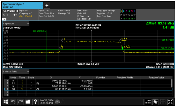
Figure 85 - 802.11ax HE80 SU LPI Minimum 99% OBW
