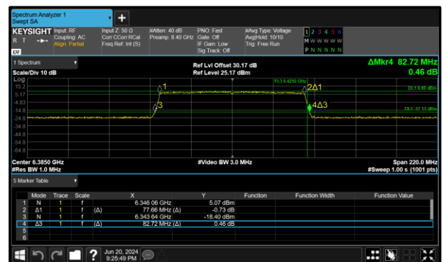
Figure 84 - 802.11ax HE80 SU SP Maximum 99% OBW
