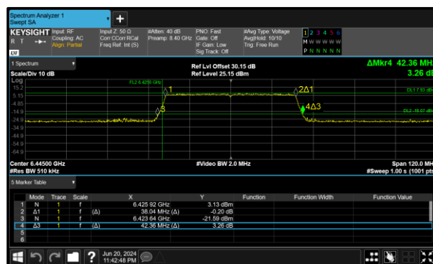
Figure 156 - 802.11ax HE40 SU SP Maximum 26 dB EBW
