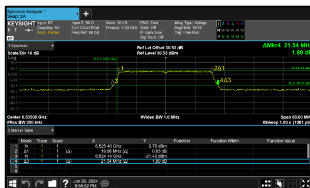
Figure 154 - 802.11ax HE20 SU SP Maximum 26 dB EBW
