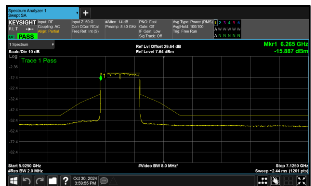
Figure 336 - A (Core 0) 802.11ax HE160 SU LPI 6345 MHz (CH79)
