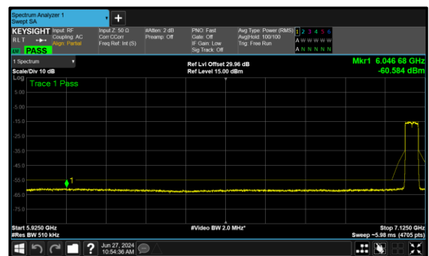
Figure 334 - B (Core 1) 802.11ax HE40 SU LPI 7085 MHz (CH227)
