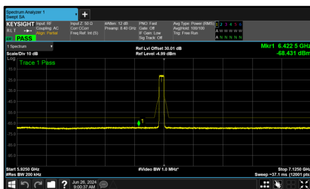
Figure 317 - A (Core 0) 802.11ax HE20 SU LPI 6515 MHz (CH113)
