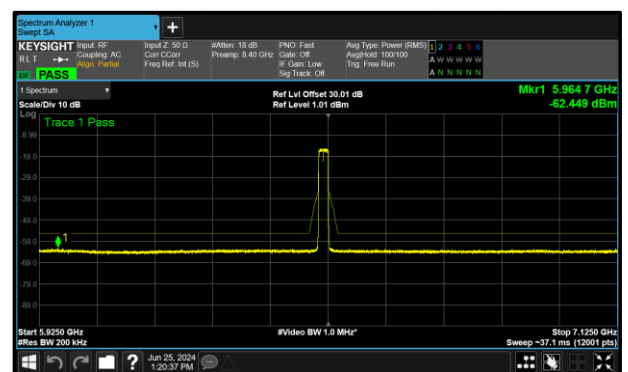
Figure 296 - A (Core 0) 802.11ax HE20 SU LPI 6515 MHz (CH113)
