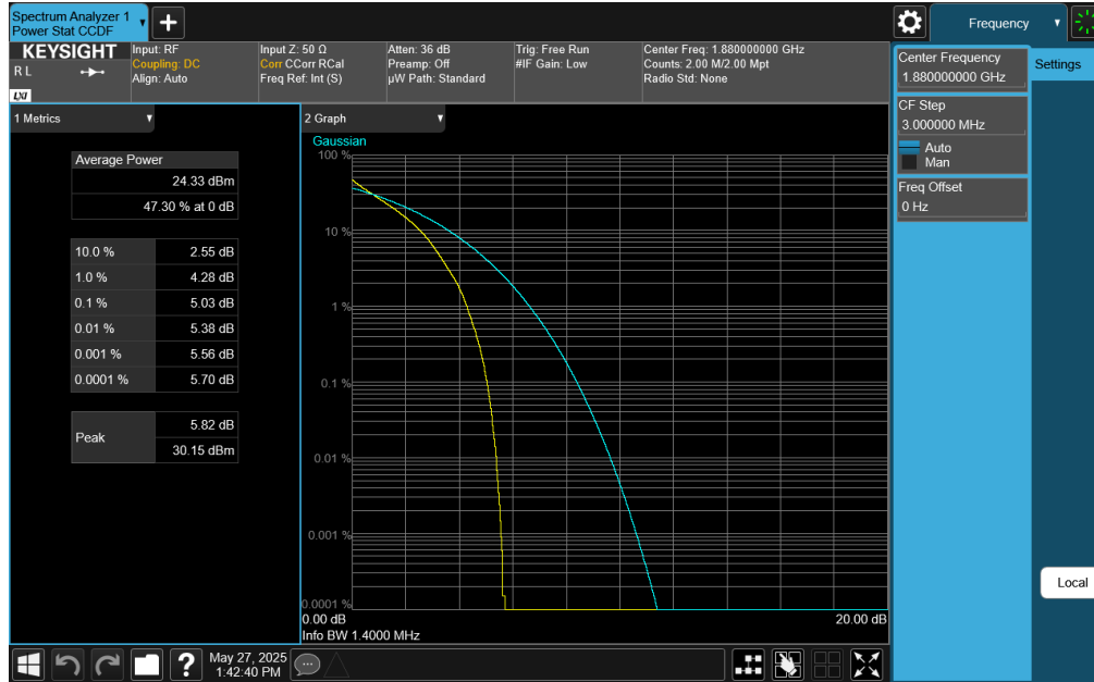
Plot 7-233. PAR Plot (LTE Band 2 - 1.4MHz QPSK - Full RB Configuration)
