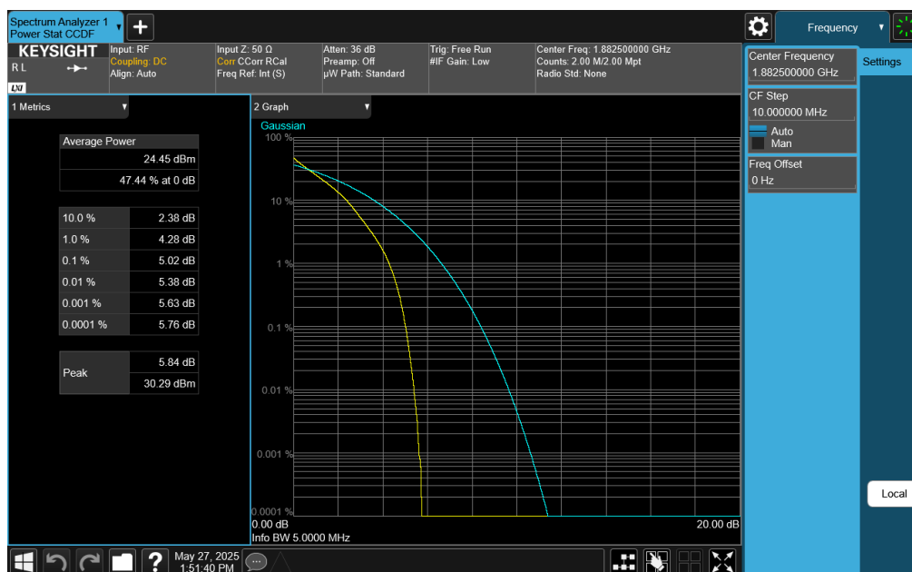
Plot 7-217. PAR Plot (LTE Band 25 - 5MHz QPSK - Full RB Configuration)
