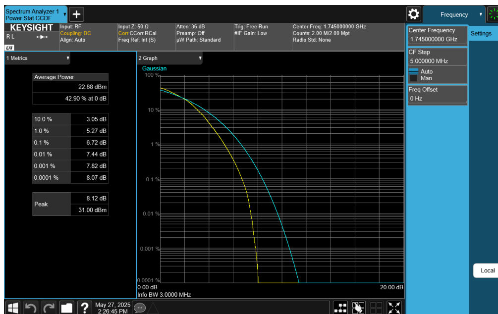
Plot 7-389. PAR Plot (LTE Band 66 - 3MHz 64-QAM - Full RB)
