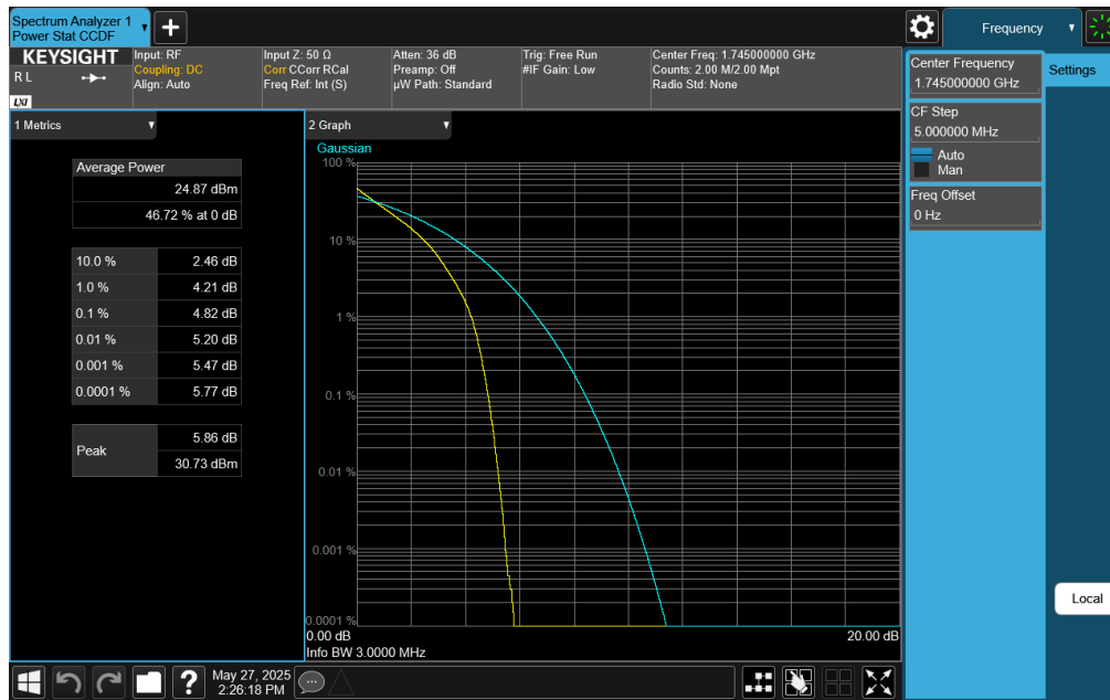
Plot 7-387. PAR Plot (LTE Band 66 - 3MHz QPSK - Full RB)
