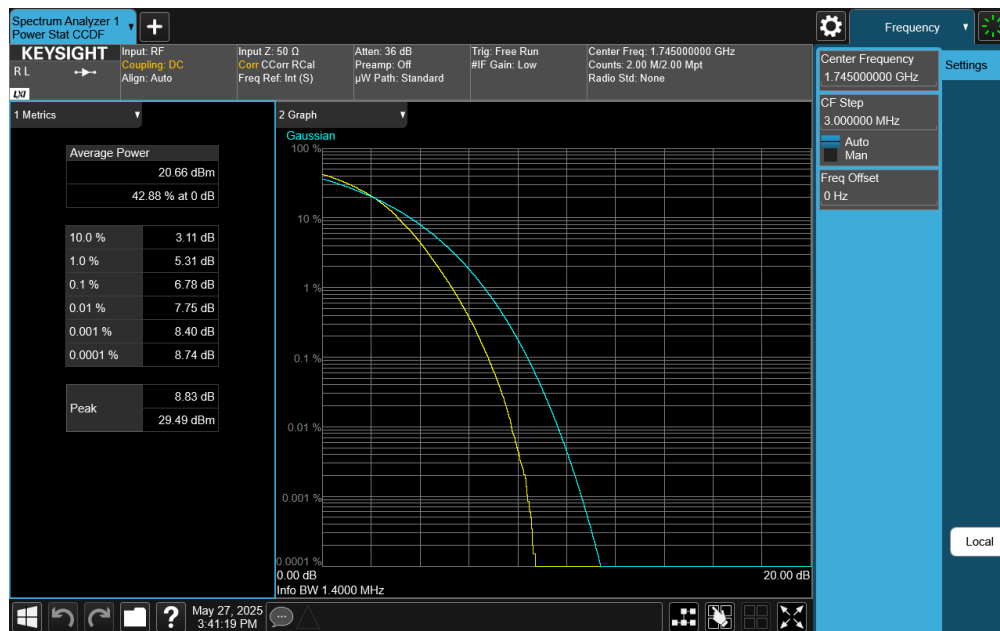
Plot 7-386. PAR Plot (LTE Band 66 - 1.4MHz 256-QAM - Full RB)
