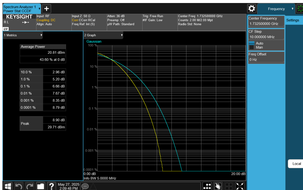
Plot 7-418. PAR Plot (LTE Band 4 - 5MHz 256-QAM - Full RB)
