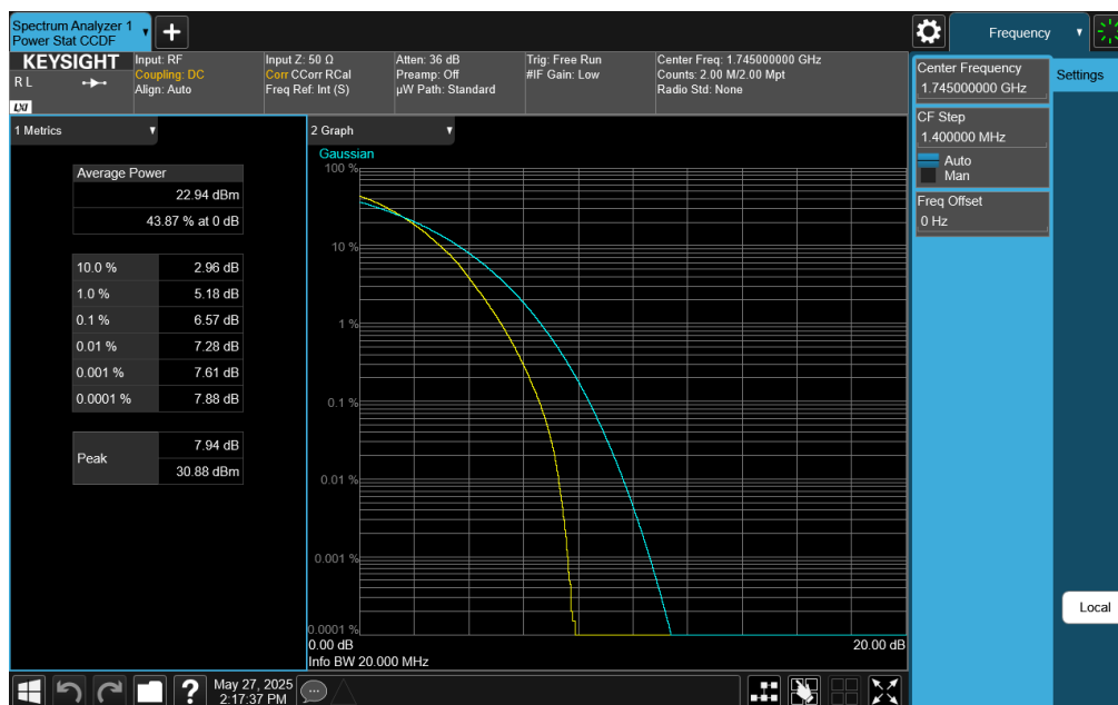
Plot 7-405. PAR Plot (LTE Band 66 - 20MHz 64-QAM - Full RB)
