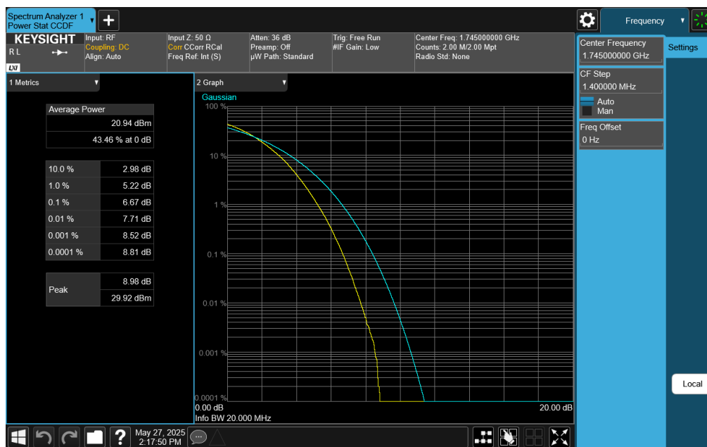
Plot 7-406. PAR Plot (LTE Band 66 - 20MHz 256-QAM - Full RB)
