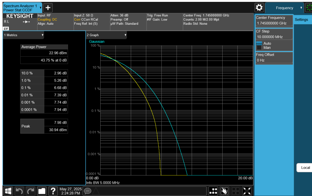
Plot 7-393. PAR Plot (LTE Band 66 - 5MHz 64-QAM - Full RB)
