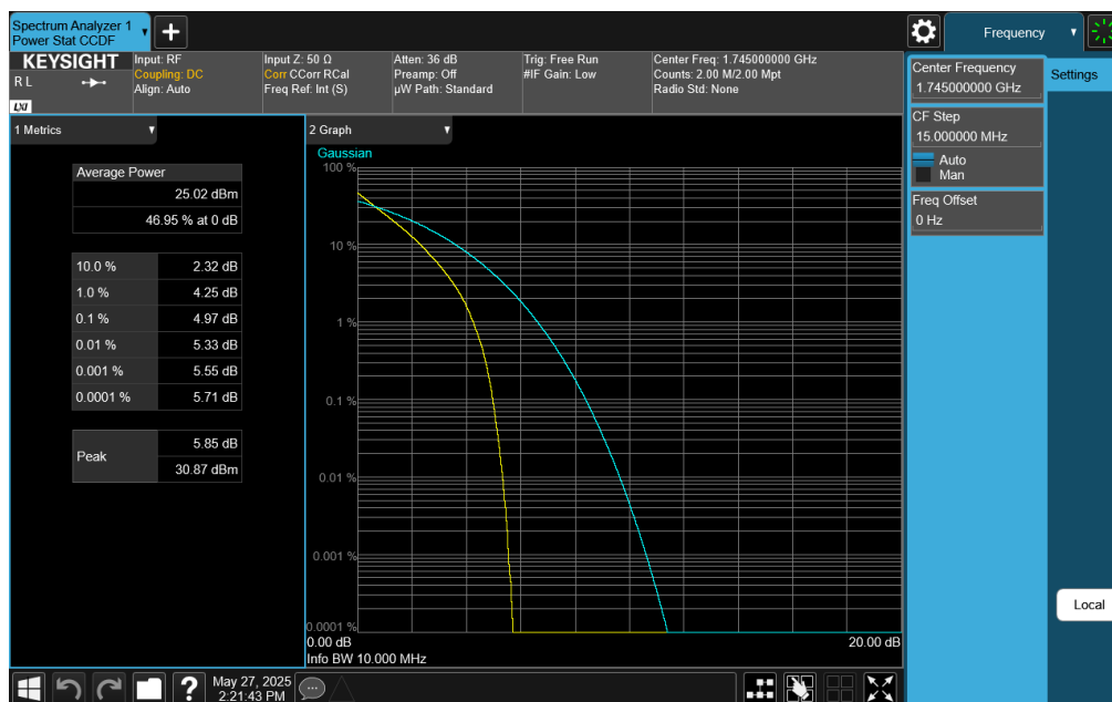
Plot 7-395. PAR Plot (LTE Band 66 - 10MHz QPSK - Full RB)
