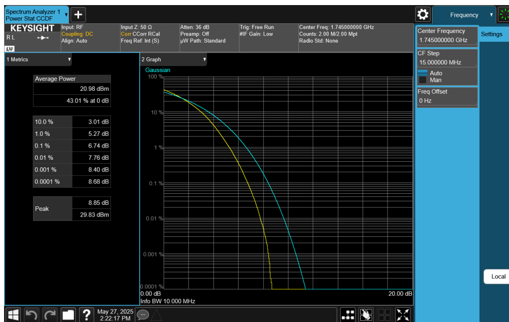
Plot 7-398. PAR Plot (LTE Band 66 - 10MHz 256-QAM - Full RB)
