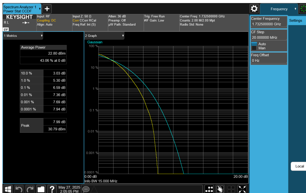
Plot 7-425. PAR Plot (LTE Band 4 - 15MHz 64-QAM - Full RB)
