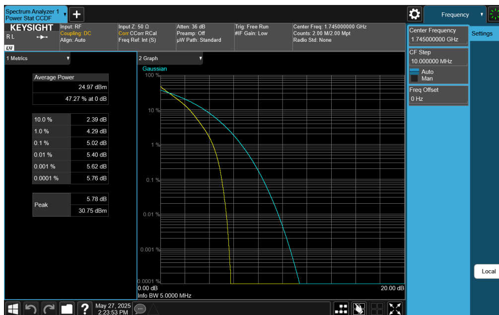
Plot 7-391. PAR Plot (LTE Band 66 - 5MHz QPSK - Full RB)
