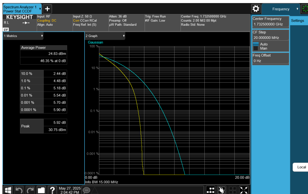
Plot 7-423. PAR Plot (LTE Band 4 - 15MHz QPSK - Full RB)
