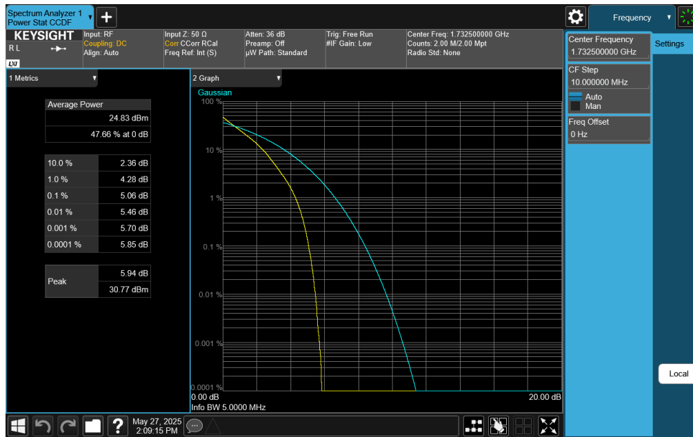
Plot 7-415. PAR Plot (LTE Band 4 - 5MHz QPSK - Full RB)
