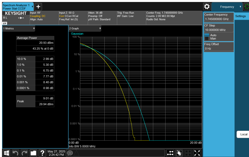
Plot 7-394. PAR Plot (LTE Band 66 - 5MHz 256-QAM - Full RB)
