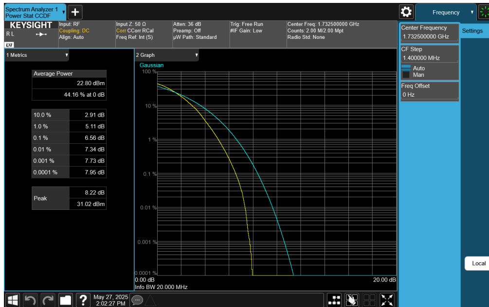
Plot 7-429. PAR Plot (LTE Band 4 - 20MHz 64-QAM - Full RB)
