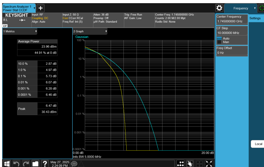
Plot 7-392. PAR Plot (LTE Band 66 - 5MHz 16-QAM - Full RB)
