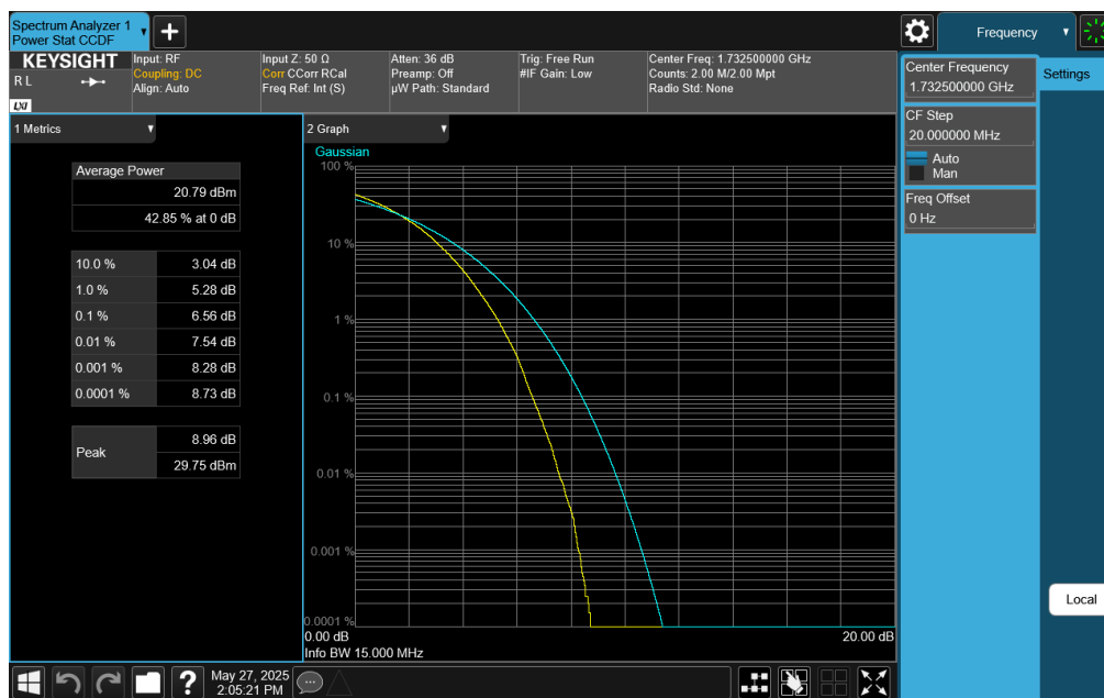
Plot 7-426. PAR Plot (LTE Band 4 - 15MHz 256-QAM - Full RB)
