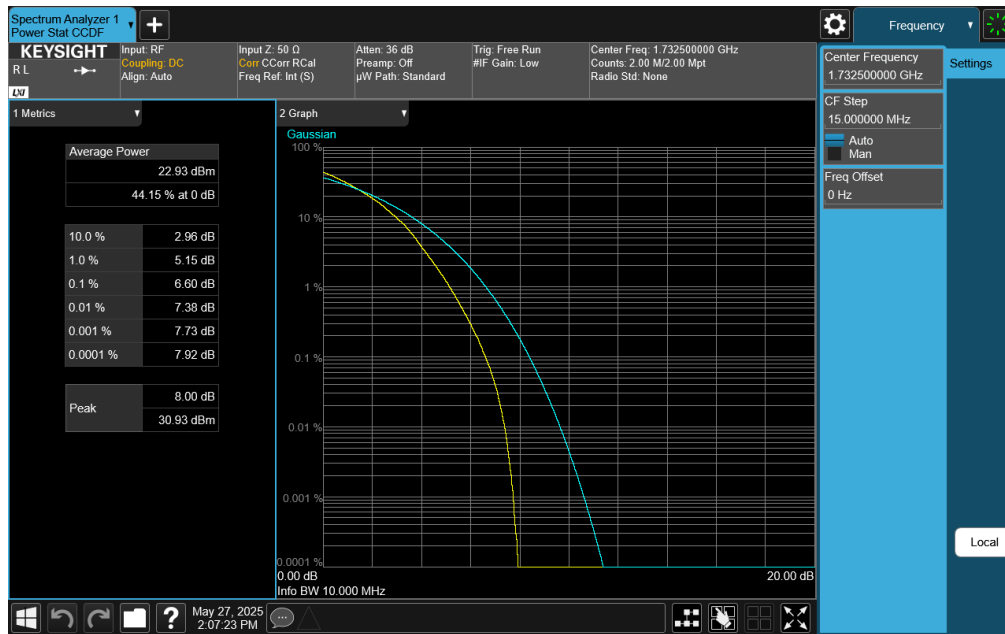
Plot 7-421. PAR Plot (LTE Band 4 - 10MHz 64-QAM - Full RB)
