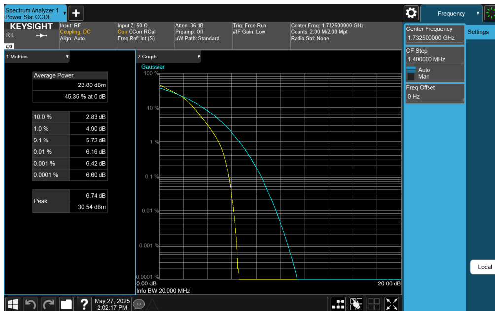
Plot 7-428. PAR Plot (LTE Band 4 - 20MHz 16-QAM - Full RB)
