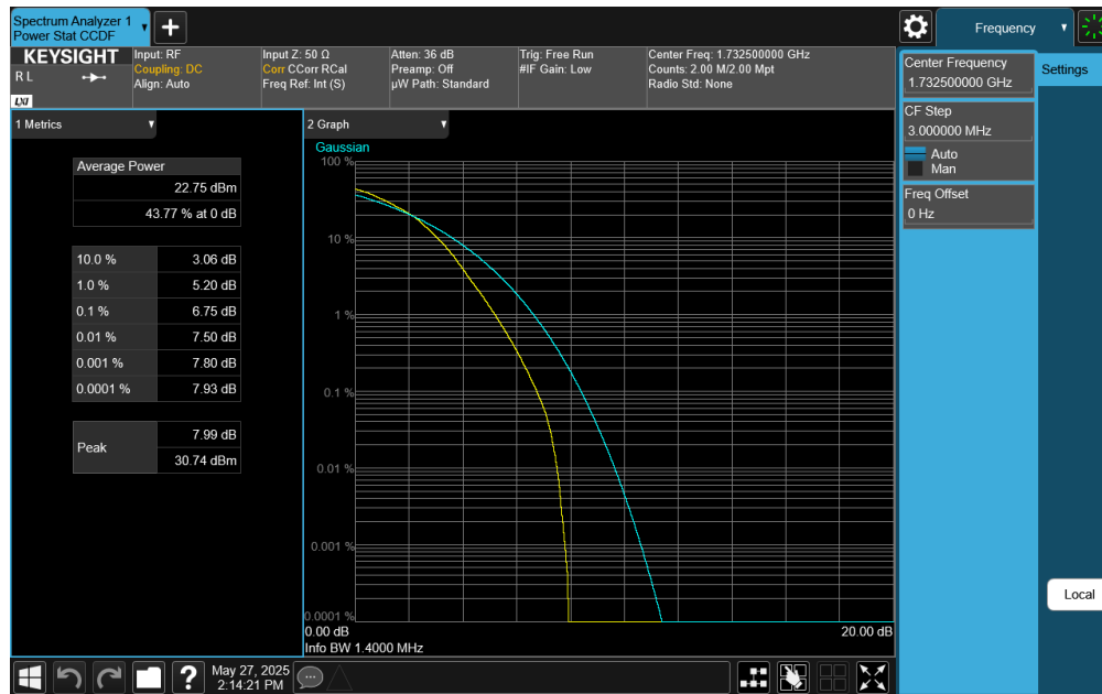
Plot 7-409. PAR Plot (LTE Band 4 - 1.4MHz 64-QAM - Full RB)
