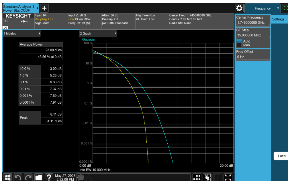
Plot 7-397. PAR Plot (LTE Band 66 - 10MHz 64-QAM - Full RB)
