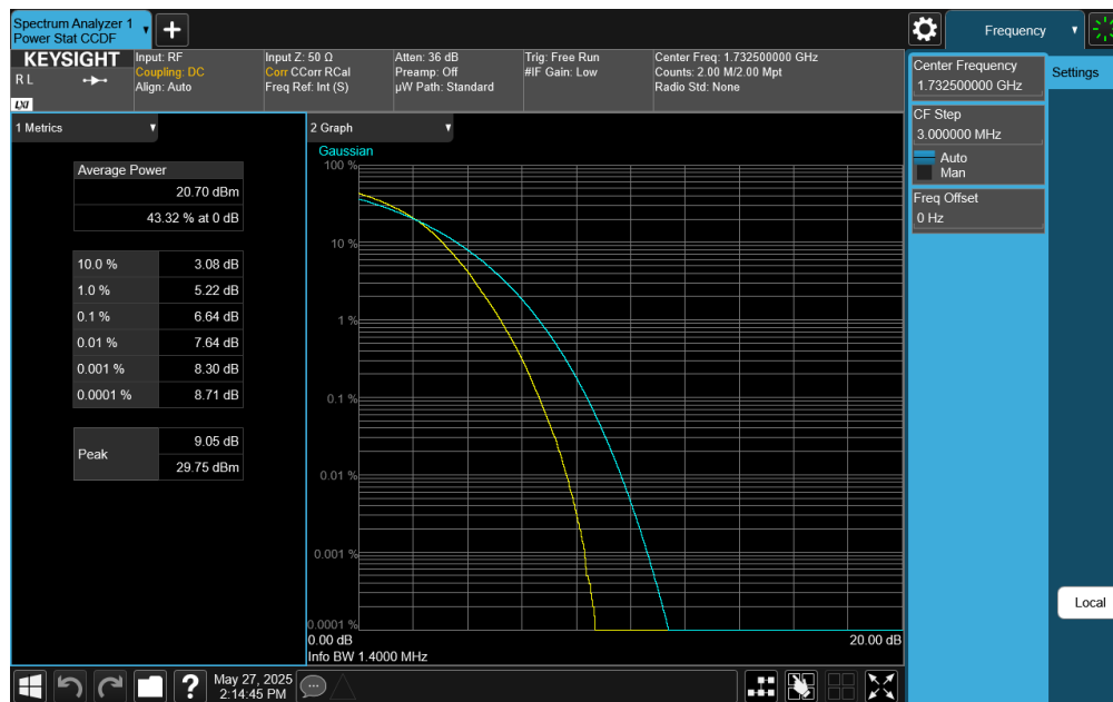
Plot 7-410. PAR Plot (LTE Band 4 - 1.4MHz 256-QAM - Full RB)
