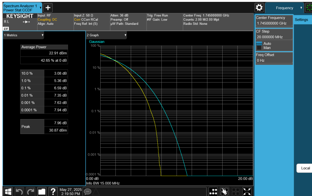
Plot 7-401. PAR Plot (LTE Band 66 - 15MHz 64-QAM - Full RB)
