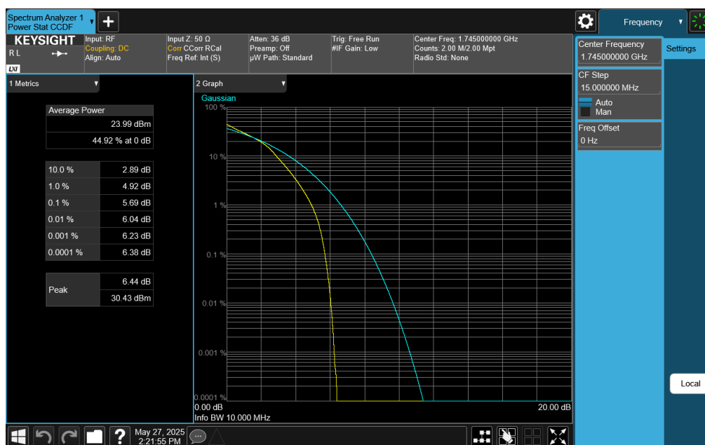
Plot 7-396. PAR Plot (LTE Band 66 - 10MHz 16-QAM - Full RB)
