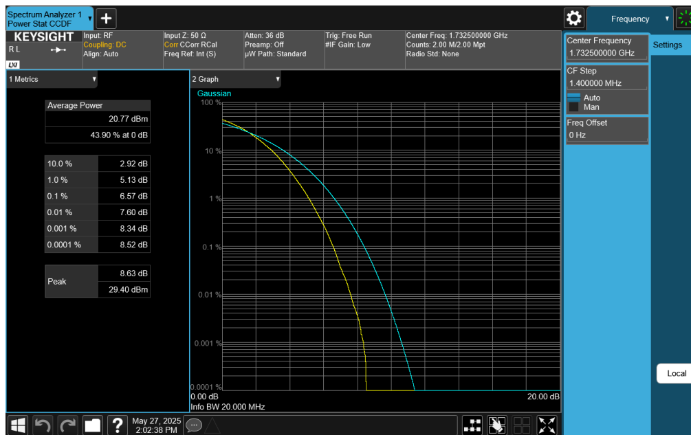
Plot 7-430. PAR Plot (LTE Band 4 - 20MHz 256-QAM - Full RB)
