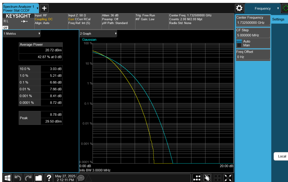
Plot 7-414. PAR Plot (LTE Band 4 - 3MHz 256-QAM - Full RB)
