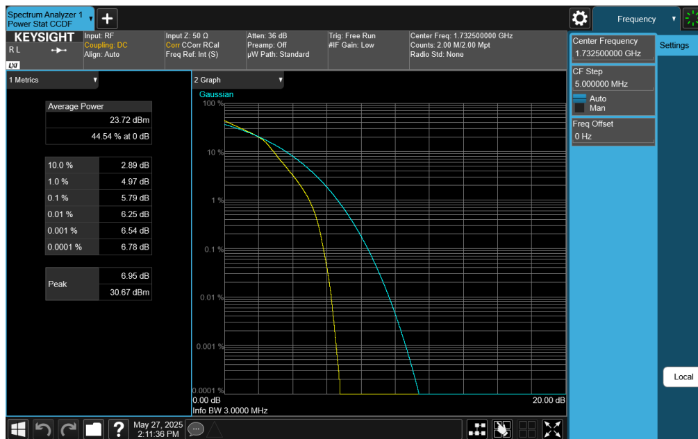
Plot 7-412. PAR Plot (LTE Band 4 - 3MHz 16-QAM - Full RB)
