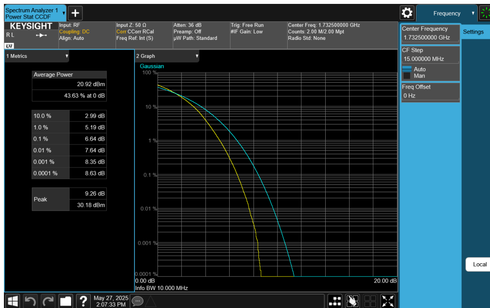
Plot 7-422. PAR Plot (LTE Band 4 - 10MHz 256-QAM - Full RB)
