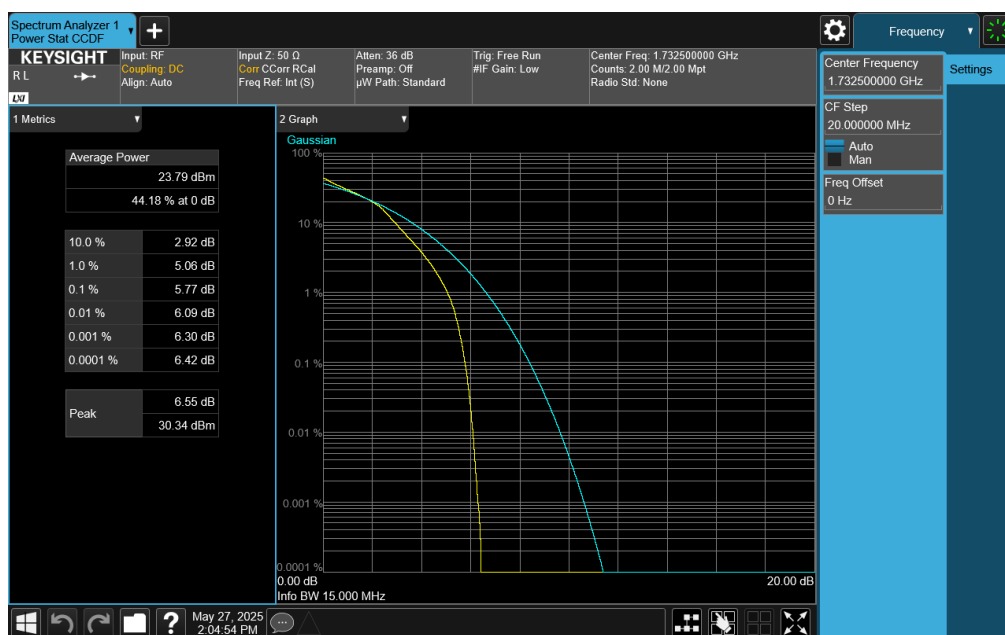
Plot 7-424. PAR Plot (LTE Band 4 - 15MHz 16-QAM - Full RB)
