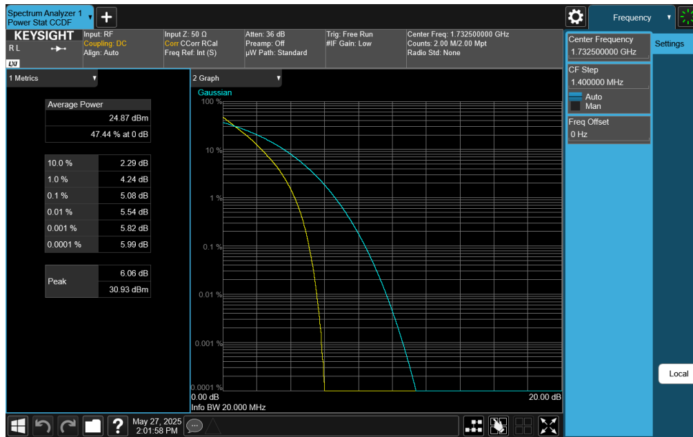
Plot 7-427. PAR Plot (LTE Band 4 - 20MHz QPSK - Full RB)
