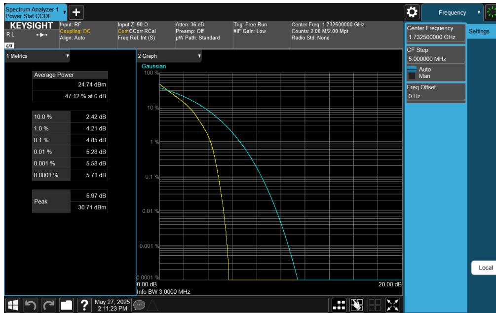
Plot 7-411. PAR Plot (LTE Band 4 - 3MHz QPSK - Full RB)
