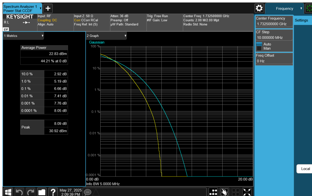
Plot 7-417. PAR Plot (LTE Band 4 - 5MHz 64-QAM - Full RB)
