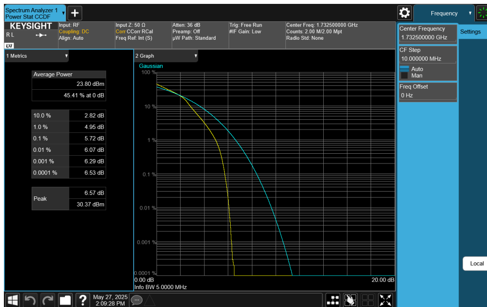
Plot 7-416. PAR Plot (LTE Band 4 - 5MHz 16-QAM - Full RB)
