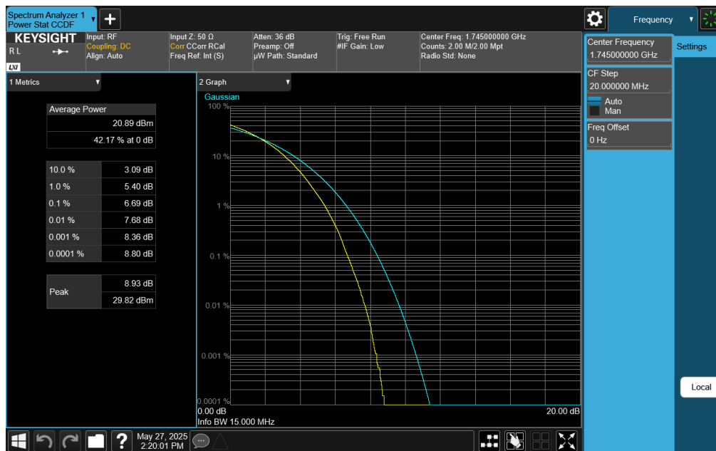
Plot 7-402. PAR Plot (LTE Band 66 - 15MHz 256-QAM - Full RB)
