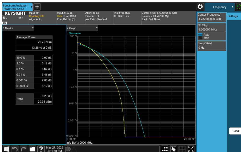
Plot 7-413. PAR Plot (LTE Band 4 - 3MHz 64-QAM - Full RB)
