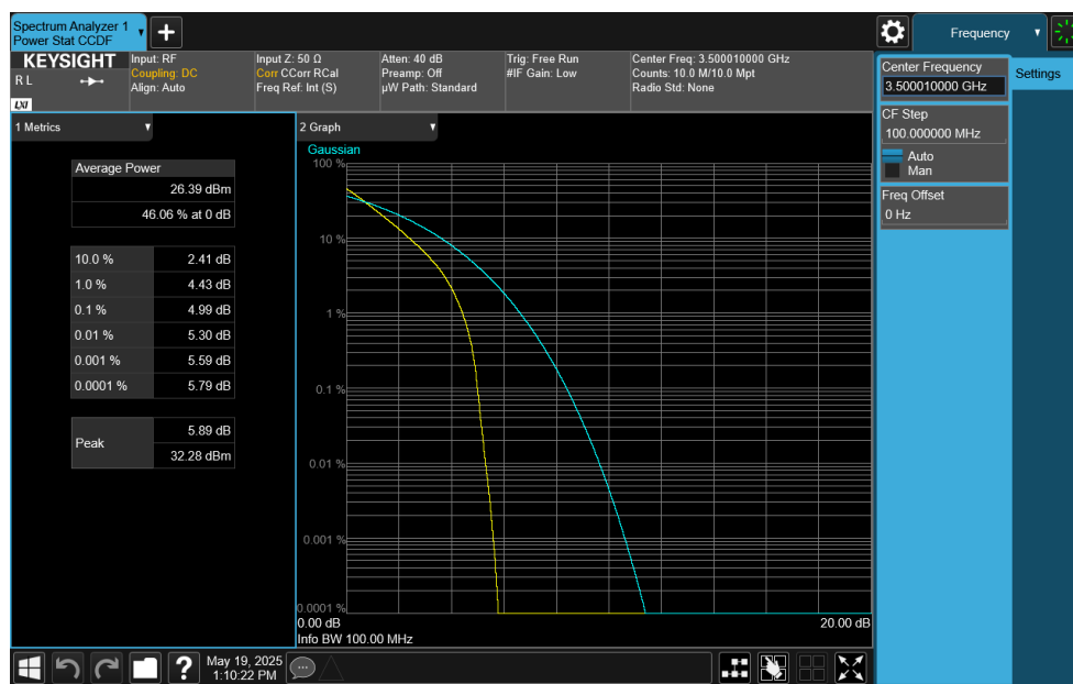
Plot 7-339. PAR Plot (NR Band n77 DoD-Band - 100MHz DFT-s-OFDM QPSK - Full RB)
