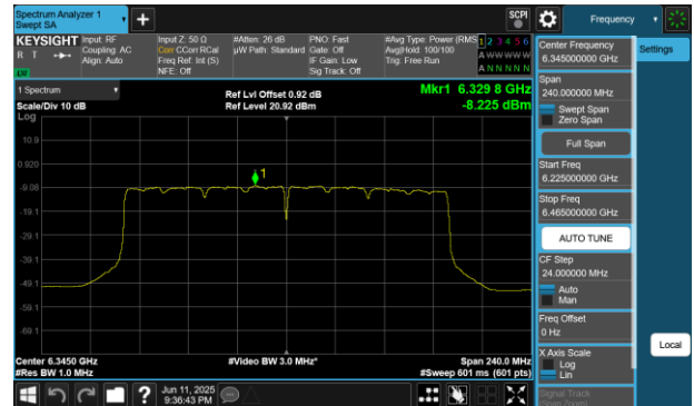
Plot 7-68 PSD Antenna 4a (160MHz BW 802.11b(SU) - Ch.79)
