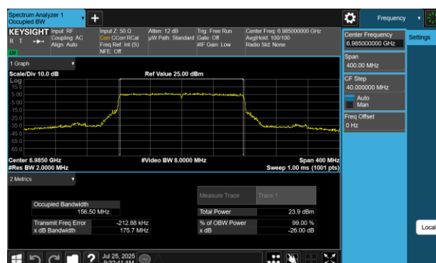
Plot 7-32 26dB BW & 99% OBW Antenna 4a (160MHz BW 802.11be(SU) - Ch.207)
