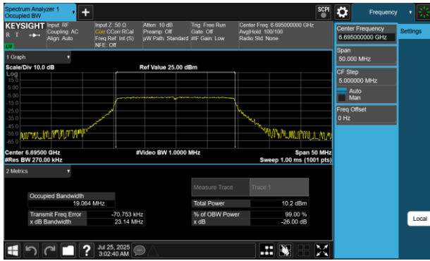
Plot 7-41 26dB BW & 99% OBW Antenna 2a (20MHz BW 802.11be(SU) - Ch.149)
