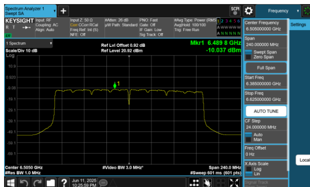
Plot 7-72 PSD Antenna 4a (160MHz BW 802.11be(SU) - Ch.111)
