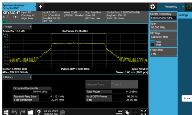
Plot 7-29 26dB BW & 99% OBW Antenna 4a (20MHz BW 802.11be(SU) - Ch.189)
