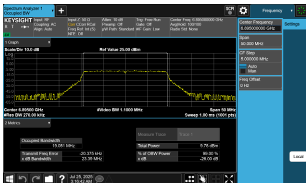
Plot 7-45 26dB BW & 99% OBW Antenna 2a (20MHz BW 802.11be(SU) - Ch.189)
