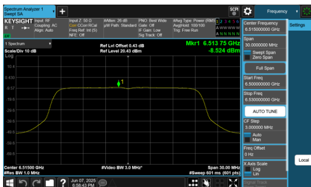
Plot 7-53 PSD Antenna WF5B (20MHz BW 802.11be(SU) - Ch.113)
