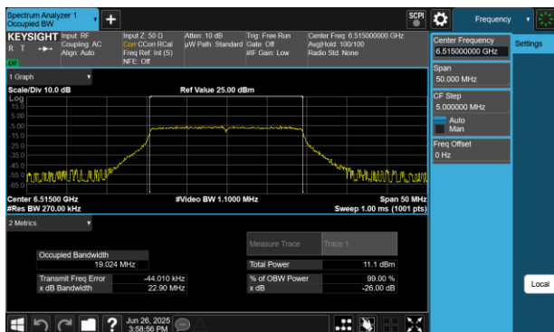
Plot 7-21 26dB BW & 99% OBW Antenna 4a (20MHz BW 802.11be(SU) - Ch.113)
