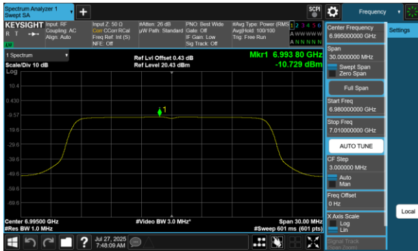
Plot 7-61 PSD Antenna WF5B (20MHz BW 802.11be(SU) - Ch.209)
