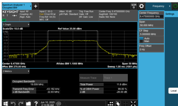
Plot 7-37 26dB BW & 99% OBW Antenna 2a (20MHz BW 802.11be(SU) - Ch.105)
