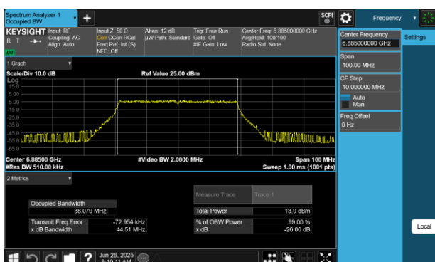
Plot 7-46 26dB BW & 99% OBW Antenna 2a (40MHz BW 802.11be(SU) - Ch.187)
