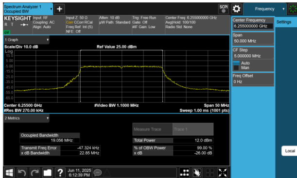
Plot 7-17 26dB BW & 99% OBW Antenna 4a (20MHz BW 802.11be(SU) - Ch.61)
