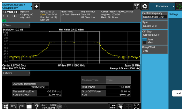
Plot 7-25 26dB BW & 99% OBW Antenna 4a (20MHz BW 802.11be(SU) - Ch.185)
