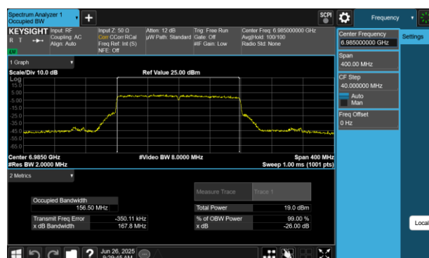
Plot 7-48 26dB BW & 99% OBW Antenna 2a (160MHz BW 802.11be(SU) - Ch.207)
