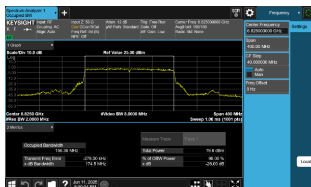
Plot 7-28 26dB BW & 99% OBW Antenna 4a (160MHz BW 802.11be(SU) - Ch.175)
