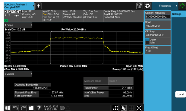
Plot 7-72 26dB BW & 99% OBW Antenna 2a (160MHz BW 802.11be(SU) - Ch.79)
