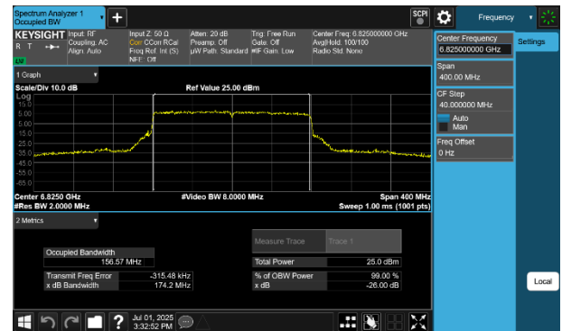
Plot 7-52 26dB BW & 99% OBW Antenna 4a (160MHz BW 802.11be(SU) - Ch.175)
