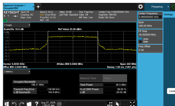
Plot 7-68 26dB BW & 99% OBW Antenna 2a (160MHz BW 802.11be(SU) - Ch.143)
