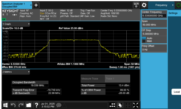
Plot 7-49 26dB BW & 99% OBW Antenna 4a (20MHz BW 802.11be(SU) - Ch.117)
