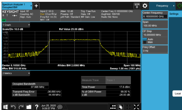
Plot 7-70 26dB BW & 99% OBW Antenna 2a (40MHz BW 802.11be(SU) - Ch.43)
