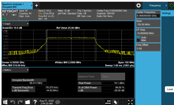
Plot 7-50 26dB BW & 99% OBW Antenna 4a (40MHz BW 802.11be(SU) - Ch.123)
