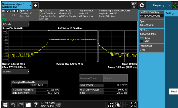
Plot 7-69 26dB BW & 99% OBW Antenna 2a (20MHz BW 802.11be(SU) - Ch.45)
