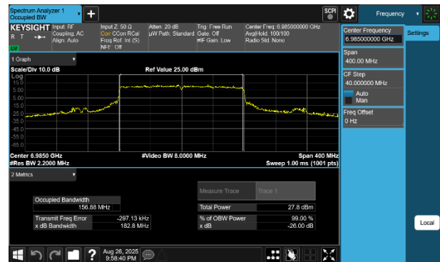
Plot 7-56 26dB BW & 99% OBW Antenna 4a (160MHz BW 802.11be(SU) - Ch.207)
