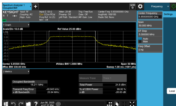
Plot 7-65 26dB BW & 99% OBW Antenna 2a (20MHz BW 802.11a - Ch.181)
