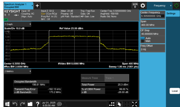
Plot 7-76 26dB BW & 99% OBW Antenna 2a (160MHz BW 802.11be(SU) - Ch.111)
