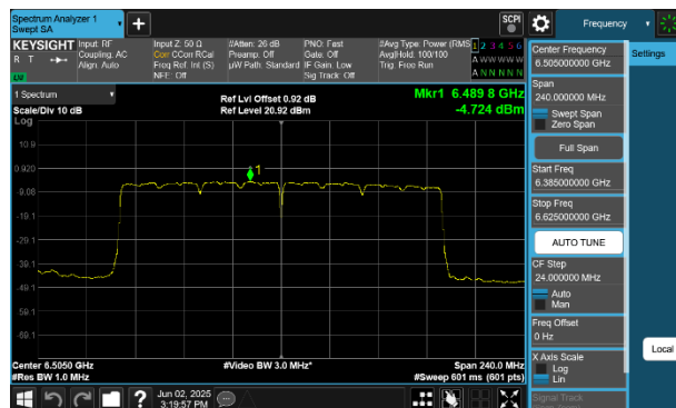
Plot 7-132 PSD Antenna 4a (160MHz BW 802.11be(SU) - Ch.111)
