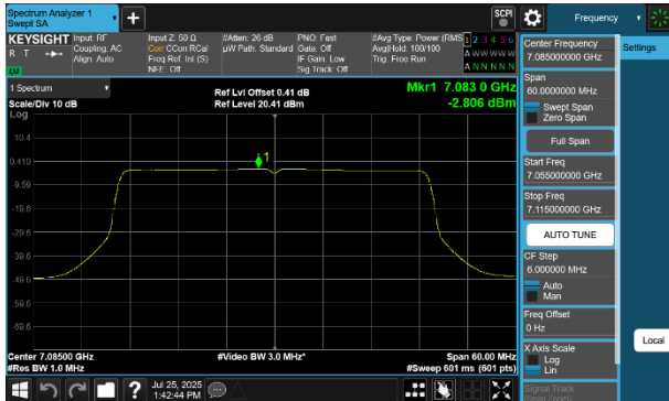
Plot 7-138 PSD Antenna 4a (40MHz BW 802.11be(SU) - Ch.227)
