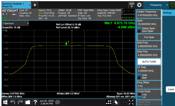
Plot 7-133 PSD Antenna 4a (20MHz BW 802.11be(SU) - Ch.185)
