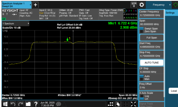
Plot 7-150 PSD Antenna 2a (40MHz BW 802.11be(SU) - Ch.155)
