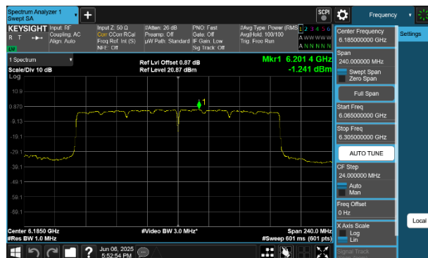
Plot 7-144 PSD Antenna 2a (160MHz BW 802.11be(SU) - Ch.47)
