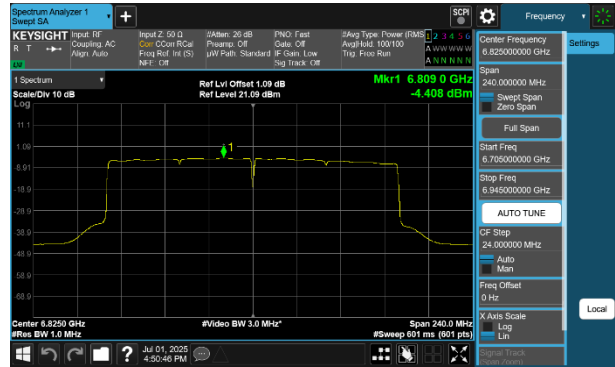
Plot 7-136 PSD Antenna 4a (160MHz BW 802.11be(SU) - Ch.175)
