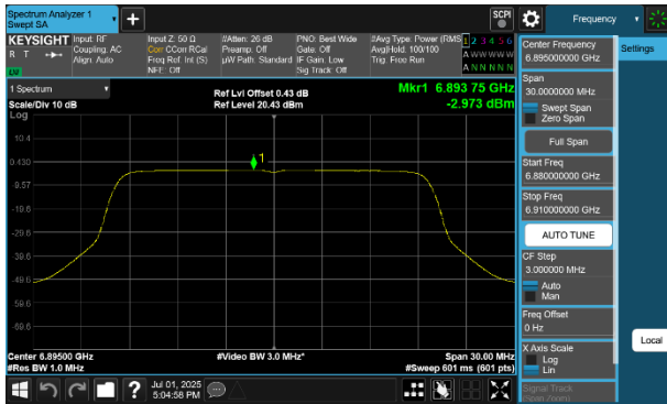
Plot 7-137 PSD Antenna 4a (20MHz BW 802.11be(SU) - Ch.189)
