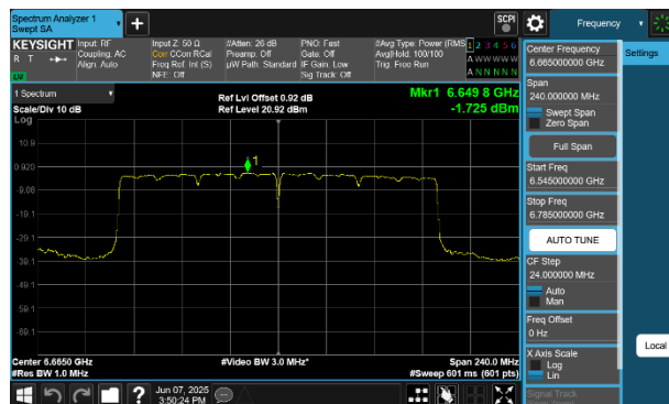
Plot 7-124 PSD Antenna 4a (160MHz BW 802.11be(SU) - Ch.143)
