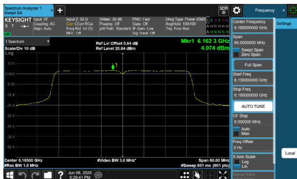
Plot 7-142 PSD Antenna 2a (40MHz BW 802.11be(SU) - Ch.43)
