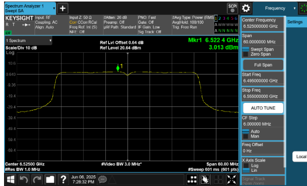
Plot 7-146 PSD Antenna 2a (40MHz BW 802.11be(SU) - Ch.115)
