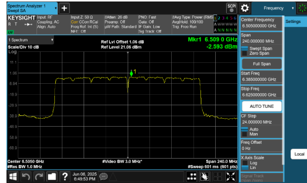
Plot 7-148 PSD Antenna 2a (160MHz BW 802.11be(SU) - Ch.111)
