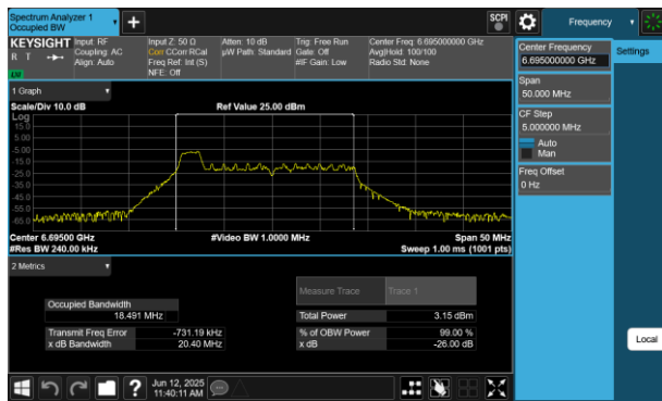
Plot 7-67 26dB BW & 99% OBW Antenna 4a (20MHz BW 802.11be(RU) RU26 Index0 - Ch.149)
