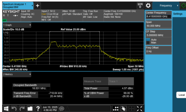
Plot 7-89 26dB BW & 99% OBW Antenna 2a (20MHz BW 802.11be(RU) RU26 Index0 - Ch.93)
