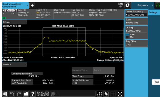
Plot 7-111 26dB BW & 99% OBW Antenna 2a (20MHz BW 802.11be(RU) RU26 Index0 - Ch.117)
