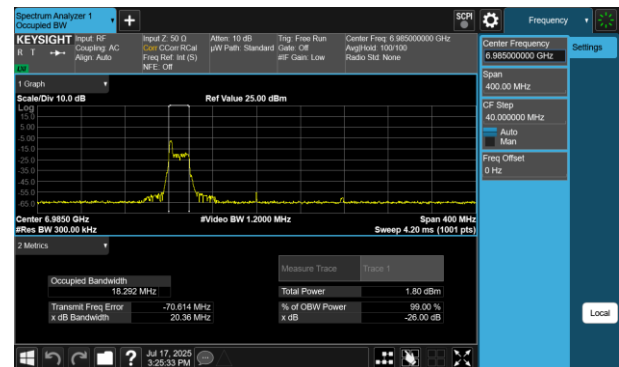
Plot 7-125 26dB BW & 99% OBW Antenna 2a (160MHz BW 802.11be(RU) RU26 Index0 - Ch.207)
