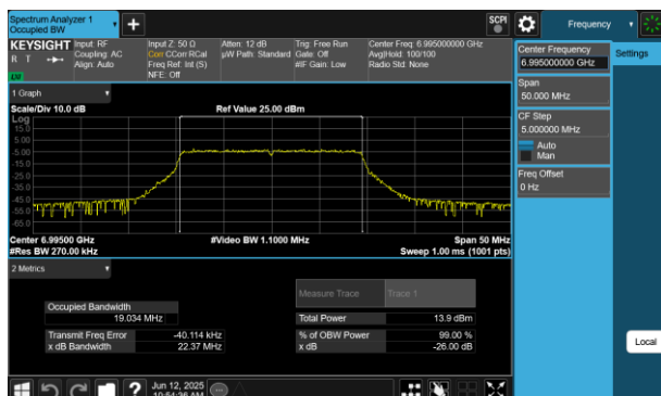
Plot 7-86 26dB BW & 99% OBW Antenna 4a (20MHz BW 802.11be(RU) RU242 Index61 - Ch.209)
