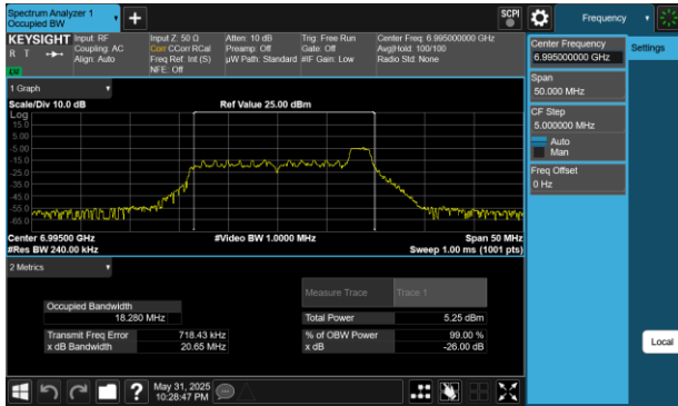
Plot 7-221 26dB BW & 99% OBW Antenna 2a (20MHz BW 802.11be(RU) RU26 Index8 - Ch.209)
