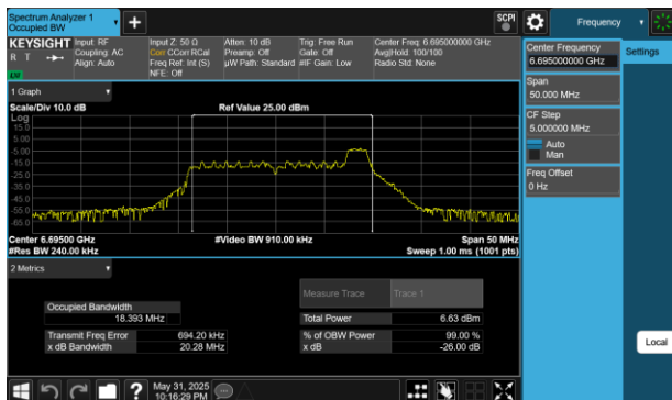
Plot 7-210 26dB BW & 99% OBW Antenna 2a (20MHz BW 802.11be(RU) RU26 Index8 - Ch.149)
