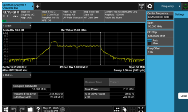
Plot 7-199 26dB BW & 99% OBW Antenna 2a (20MHz BW 802.11be(RU) RU26 Index0 - Ch.113)
