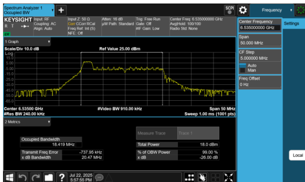
Plot 7-177 26dB BW & 99% OBW Antenna 2a (20MHz BW 802.11be(RU) RU26 Index0 - Ch.117)
