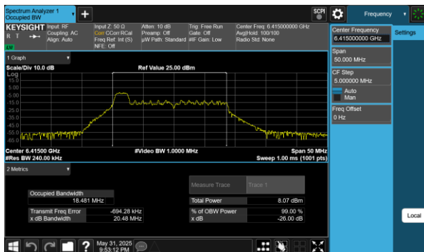
Plot 7-188 26dB BW & 99% OBW Antenna 2a (20MHz BW 802.11be(RU) RU26 Index0 - Ch.93)
