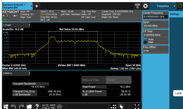
Plot 7-166 26dB BW & 99% OBW Antenna 2a (20MHz BW 802.11be(RU) RU26 Index0 - Ch.97)
