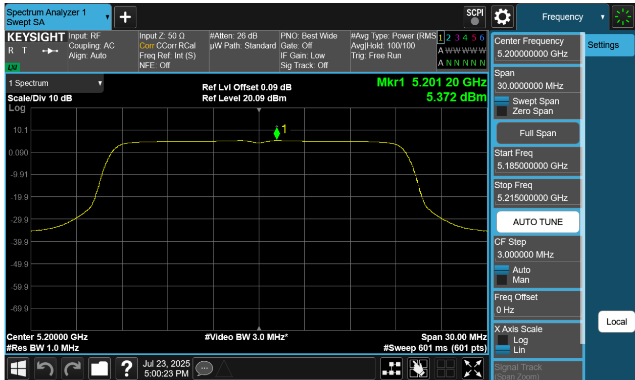
Plot 7-51 PSD Antenna 2a (20MHz BW 802.11be(SU) - Ch.40)
