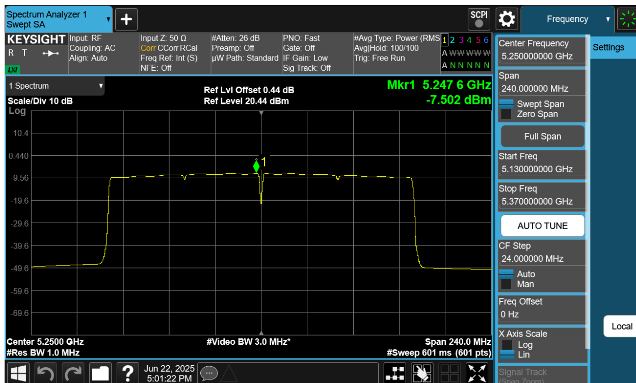
Plot 7-54 PSD Antenna 2a (160MHz BW 802.11be(SU) - Ch.50)
