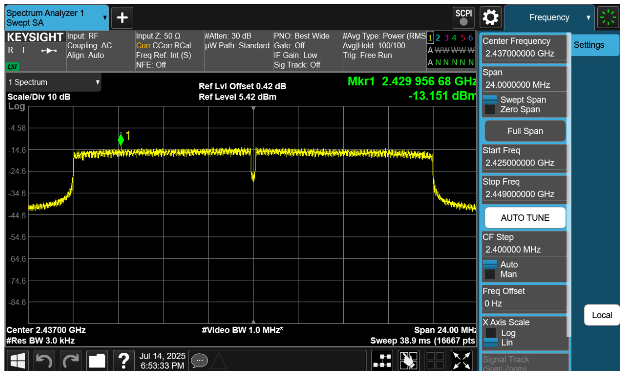
Plot 7-16 PSD Antenna 2a (20MHz BW 802.11be(SU) - Ch.6)
