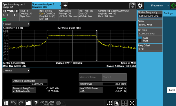
Plot 7-37 26dB BW & 99% OBW Antenna WF8 (20MHz BW 802.11be(SU) - Ch.181)
