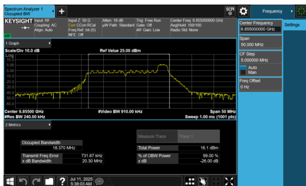
Plot 7-177 26dB BW & 99% OBW Antenna WF7 (20MHz BW 802.11be(RU) RU26 Index8 - Ch.181)
