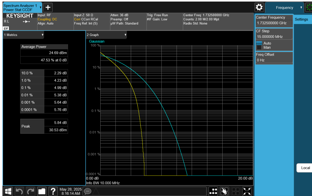
Plot 7-419. PAR Plot (LTE Band 4 - 10MHz QPSK - Full RB)
