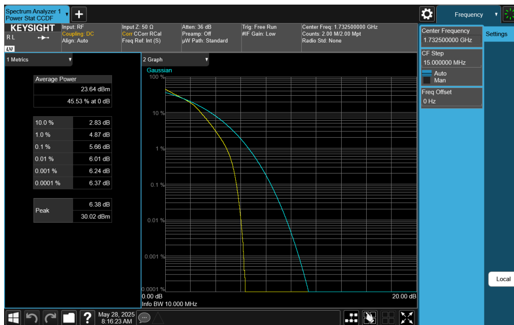
Plot 7-420. PAR Plot (LTE Band 4 - 10MHz 16-QAM - Full RB)
