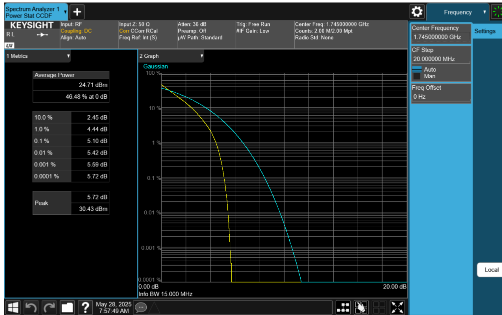
Plot 7-399. PAR Plot (LTE Band 66 - 15MHz QPSK - Full RB)
