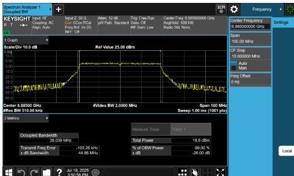
Plot 7-54 26dB BW & 99% OBW Antenna 4a (40MHz BW 802.11be(SU) - Ch.187)
