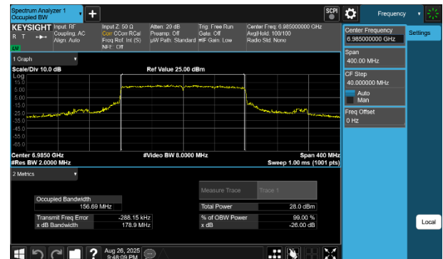
Plot 7-56 26dB BW & 99% OBW Antenna 4a (160MHz BW 802.11be(SU) - Ch.207)
