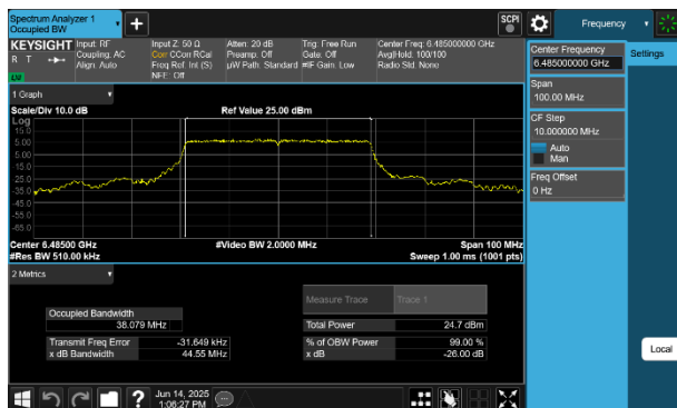
Plot 7-62 26dB BW & 99% OBW Antenna 2a (40MHz BW 802.11be(SU) - Ch.107)
