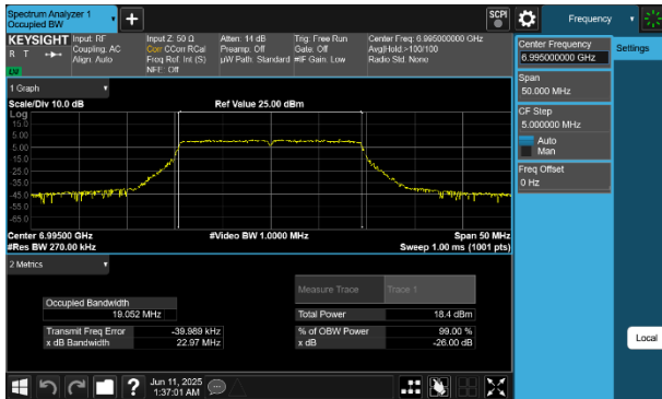
Plot 7-53 26dB BW & 99% OBW Antenna 4a (20MHz BW 802.11be(SU) - Ch.209)
