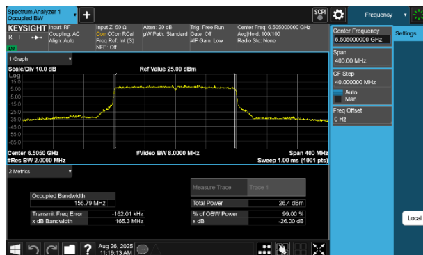
Plot 7-64 26dB BW & 99% OBW Antenna 2a (160MHz BW 802.11be(SU) - Ch.111)
