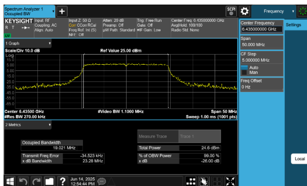
Plot 7-61 26dB BW & 99% OBW Antenna 2a (20MHz BW 802.11be(SU) - Ch.97)
