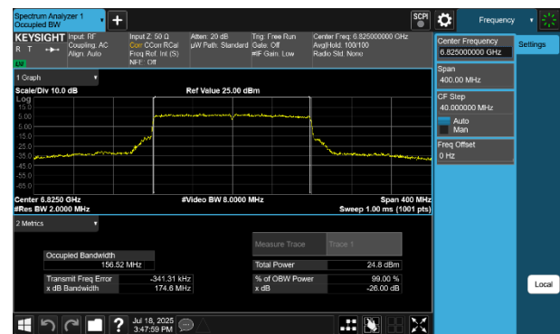
Plot 7-52 26dB BW & 99% OBW Antenna 4a (160MHz BW 802.11be(SU) - Ch.175)
