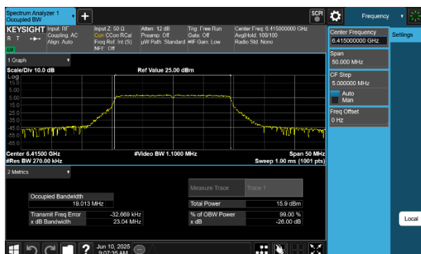
Plot 7-69 26dB BW & 99% OBW Antenna 2a (20MHz BW 802.11be(SU) - Ch.93)
