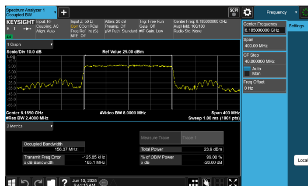
Plot 7-72 26dB BW & 99% OBW Antenna 2a (160MHz BW 802.11be(SU) - Ch.47)
