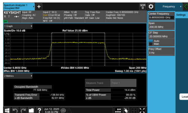
Plot 7-43 26dB BW & 99% OBW Antenna 2a (80MHz BW 802.11be(SU) - Ch.183)
