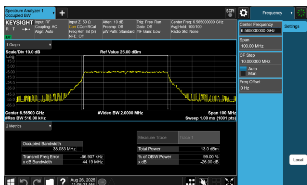
Plot 7-42 26dB BW & 99% OBW Antenna 2a (40MHz BW 802.11be(SU) - Ch.123)
