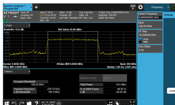
Plot 7-44 26dB BW & 99% OBW Antenna 2a (160MHz BW 802.11be(SU) - Ch.143)
