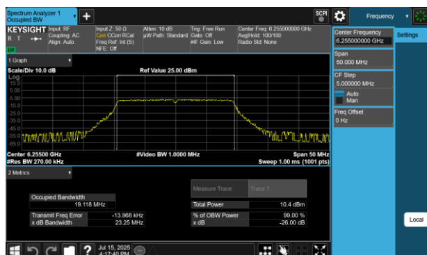
Plot 7-33 26dB BW & 99% OBW Antenna 2a (20MHz BW 802.11be(SU) - Ch.61)
