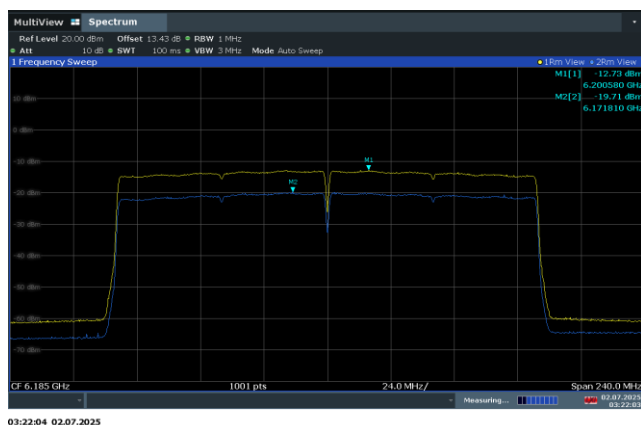
Plot 7-308. 160MHz Bandwidth – 6185MHz Antenna 4a
