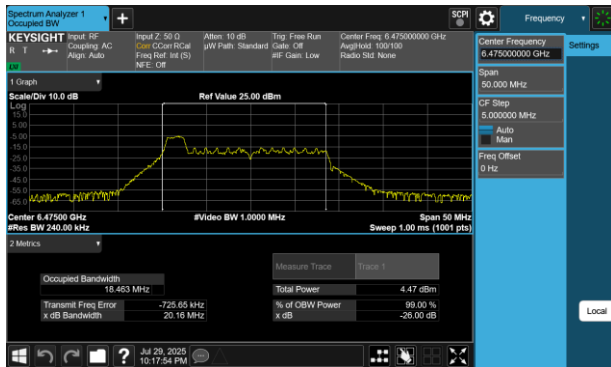
Plot 7-56 26dB BW & 99% OBW Antenna 4a (20MHz BW 802.11be(RU) RU26 Index0 - Ch.105)
