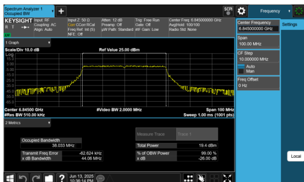
Plot 7-141 26dB BW & 99% OBW Antenna 4a(40MHz BW 802.11be(RU) RU484 Index65 - Ch.179)
