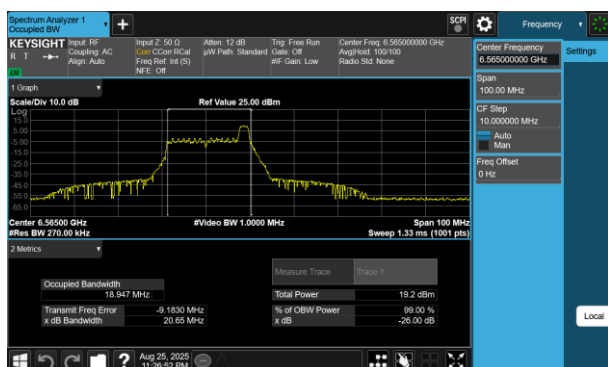
Plot 7-101 26dB BW & 99% OBW Antenna 4a(40MHz BW 802.11be(RU) RU26 Index8 - Ch.123)
