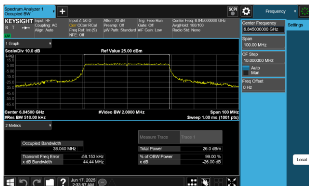
Plot 7-185 26dB BW & 99% OBW Antenna 2a (40MHz BW 802.11be(RU) RU484 Index65 - Ch.179)
