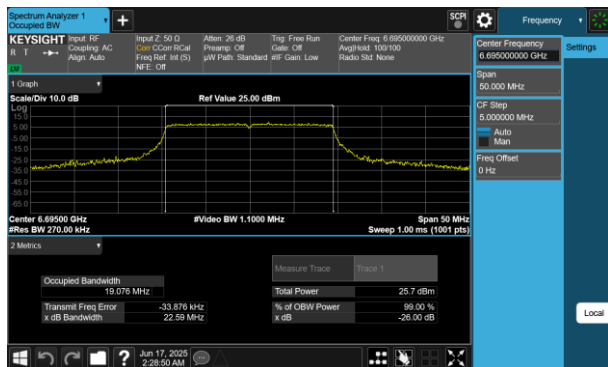
Plot 7-184 26dB BW & 99% OBW Antenna 2a (20MHz BW 802.11be(RU) RU242 Index61 - Ch.149)
