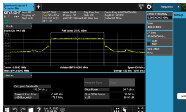
Plot 7-187 26dB BW & 99% OBW Antenna 2a (160MHz BW 802.11be(RU) RU996X2 Index68 - Ch.143)
