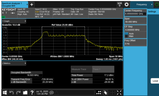
Plot 7-177 26dB BW & 99% OBW Antenna 2a (20MHz BW 802.11be(RU) RU26 Index0 - Ch.181)
