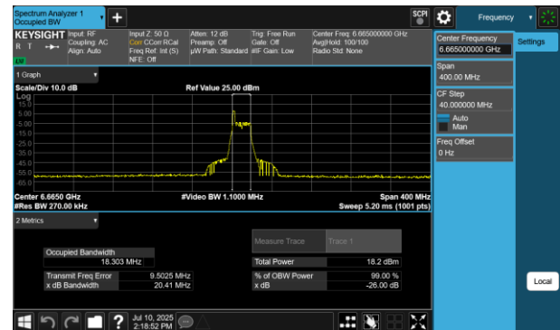
Plot 7-180 26dB BW & 99% OBW Antenna 2a (160MHz BW 802.11be(RU) RU26 Index0 - Ch.143)
