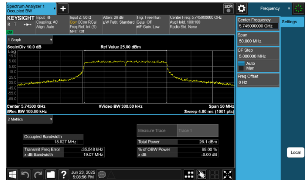
Plot 7-55 6dB BW & 99% OBW Antenna 2a (20MHz BW 802.11be(RU) RU242 Index61 - Ch.149)
