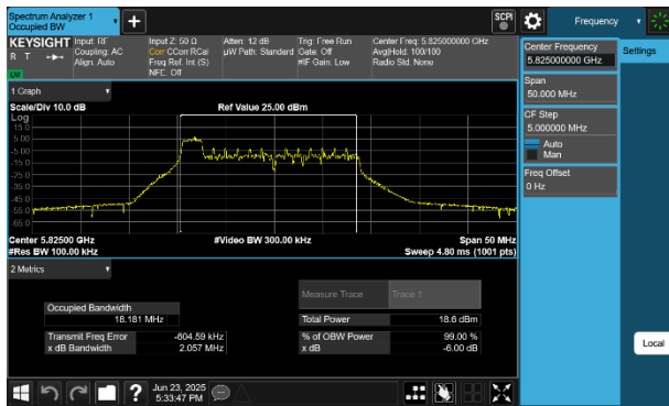
Plot 7-50 6dB BW & 99% OBW Antenna 2a (20MHz BW 802.11be(RU) RU26 Index0 - Ch.165)
