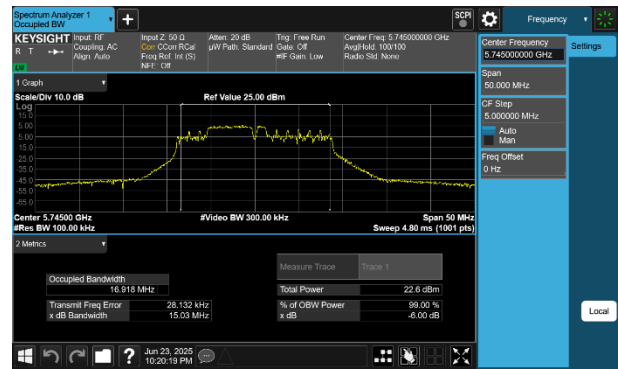
Plot 7-53 6dB BW & 99% OBW Antenna 2a (20MHz BW 802.11be(RU) RU52+26 Index71 - Ch.149)
