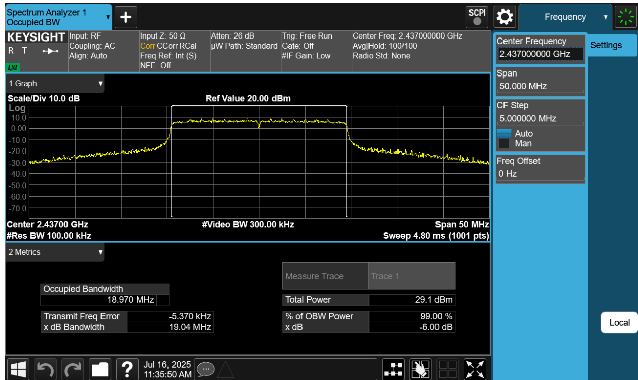
Plot 7-8 6dB BW & 99% OBW Antenna 2a (20MHz BW 802.11be(SU) - Ch.6)
