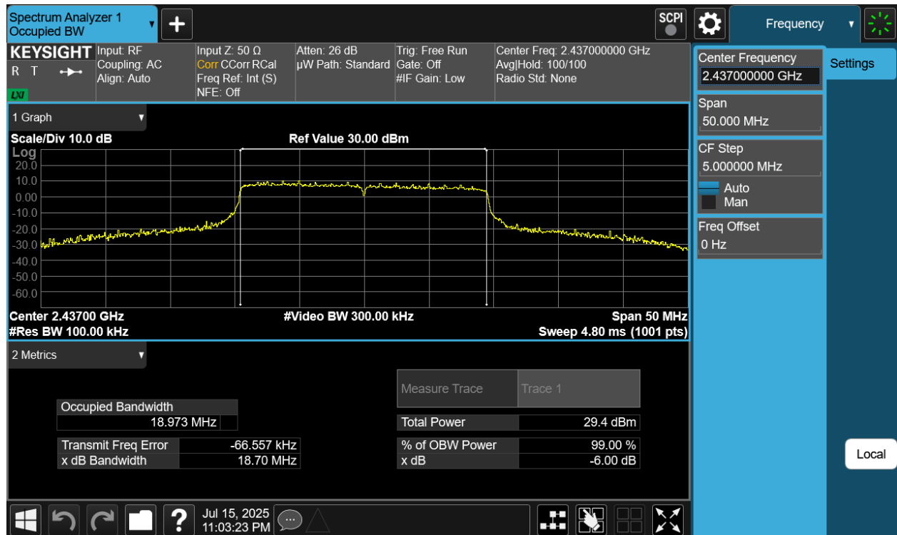
Plot 7-4 6dB BW & 99% OBW Antenna 4a (20MHz BW 802.11be(SU) - Ch.6)
