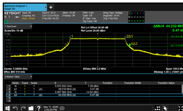
Figure 403 - 802.11ax HE40 SU Maximum 99% OBW
