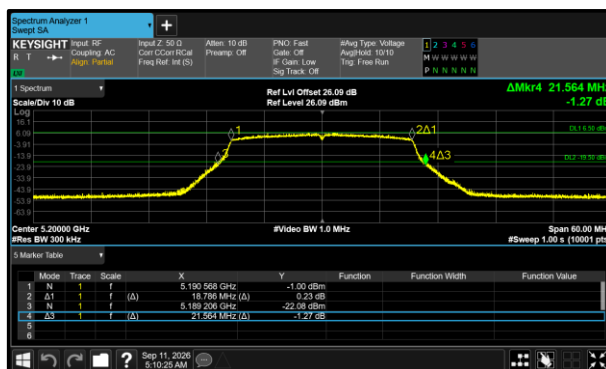
Figure 400 - 802.11ax HE20 SU Minimum 99% OBW
