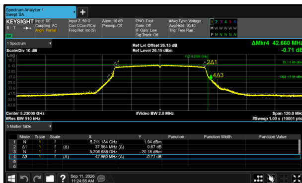
Figure 402 - 802.11ax HE40 SU Minimum 99% OBW
