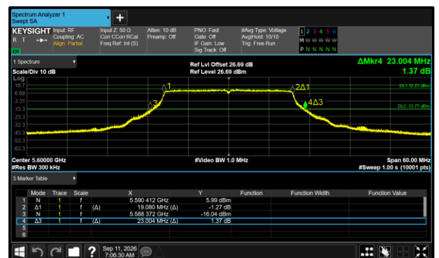
Figure 401 - 802.11ax HE20 SU Maximum 99% OBW
