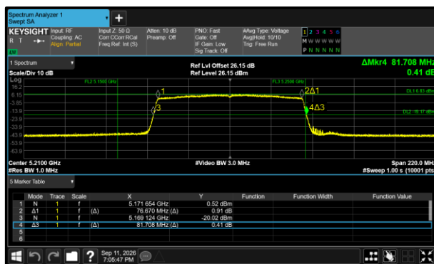
Figure 404 - 802.11ax HE80 SU Minimum 99% OBW
