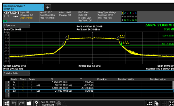
Figure 528 - 802.11ax HE20 SU Minimum 26 dB EBW
