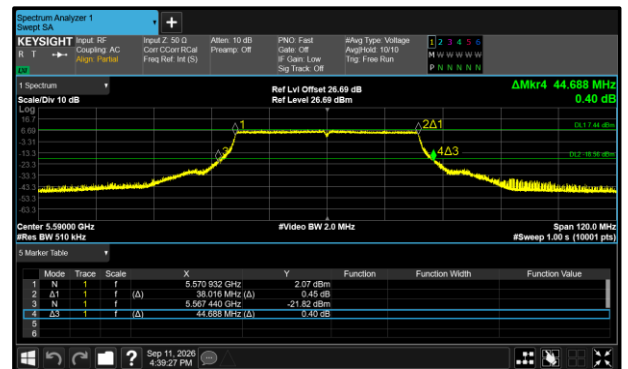
Figure 547 - 802.11ax HE40 SU Maximum 26 dB EBW
