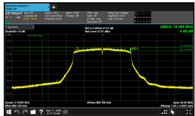
Figure 577 - 802.11ax HE20 SU Maximum 6 dB EBW
