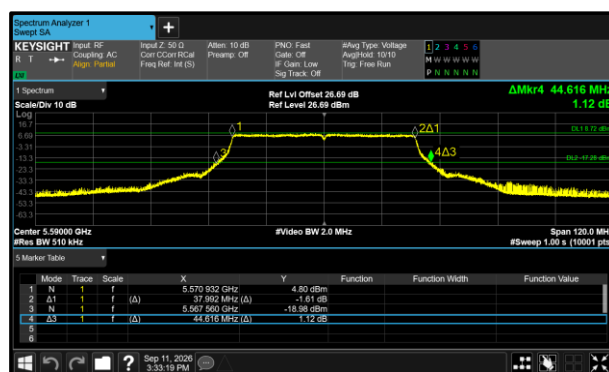
Figure 507 - 802.11ax HE40 SU Maximum 26 dB EBW
