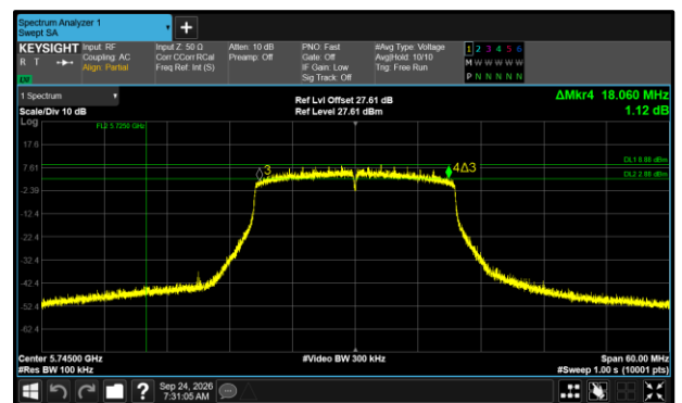
Figure 595 - 802.11ax HE20 SU Maximum 6 dB EBW
