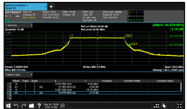
Figure 531 - 802.11ax HE40 SU Maximum 26 dB EBW
