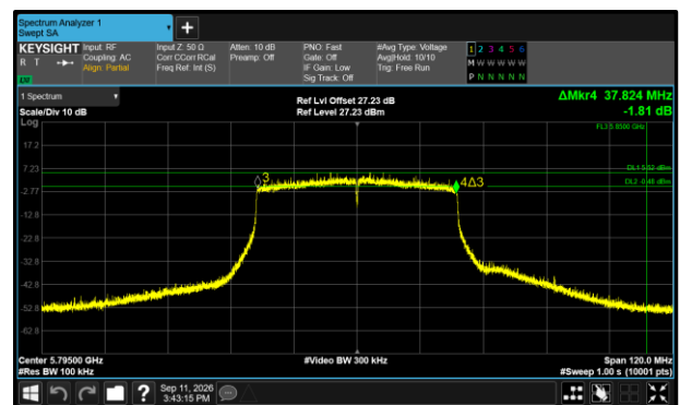
Figure 579 - 802.11ax HE40 SU Maximum 6 dB EBW
