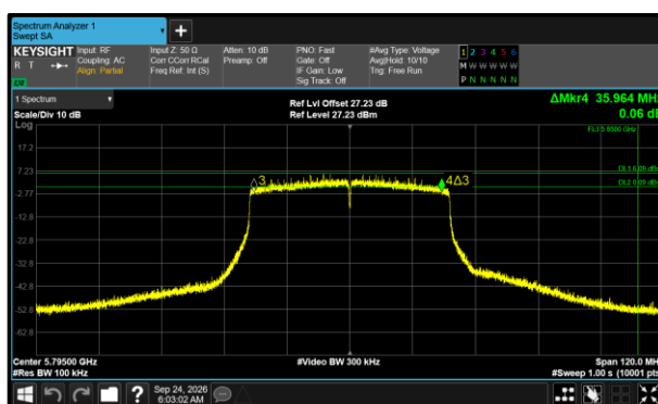
Figure 596 - 802.11ax HE40 SU Minimum 6 dB EBW
