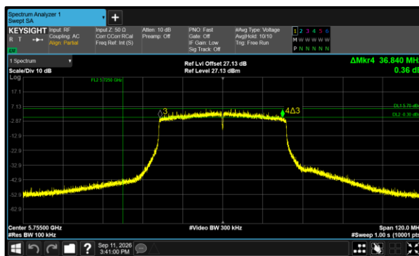
Figure 578 - 802.11ax HE40 SU Minimum 6 dB EBW
