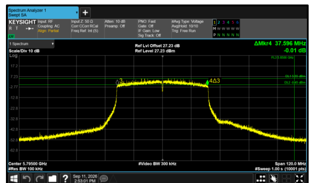
Figure 561 - 802.11ax HE40 SU Maximum 6 dB EBW
