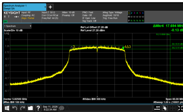
Figure 576 - 802.11ax HE20 SU Minimum 6 dB EBW
