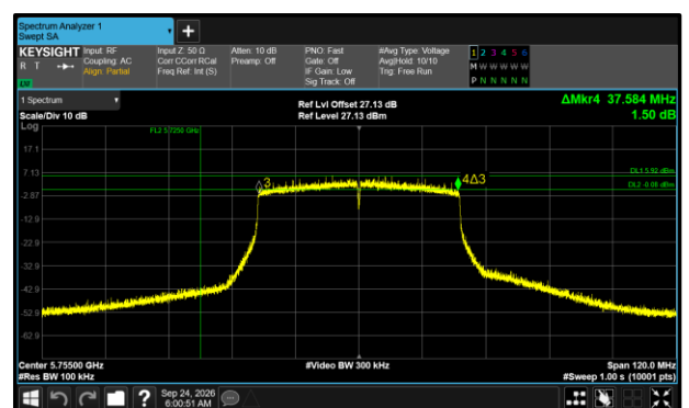
Figure 597 - 802.11ax HE40 SU Maximum 6 dB EBW
