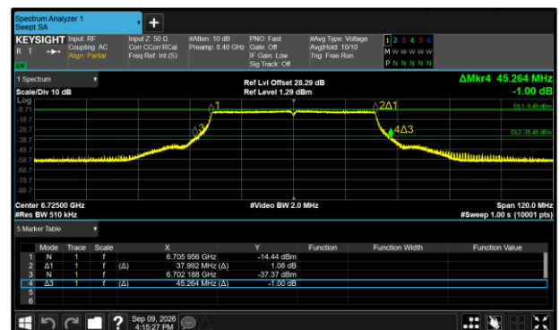
Figure 244 - 802.11ax HE40 SU LPI Maximum 26 dB EBW
