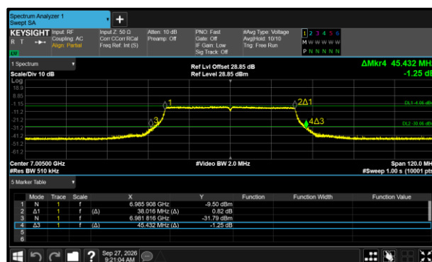
Figure 196 - 802.11ax HE40 SU LPI Maximum 26 dB EBW
