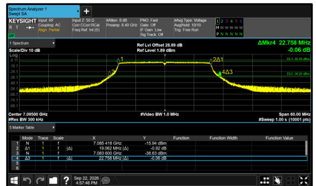
Figure 234 - 802.11ax HE20 SU VLP Maximum 99% OBW
