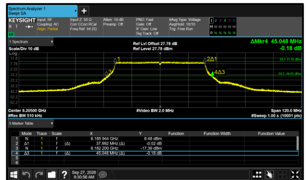
Figure 204 - 802.11ax HE40 SU SP Maximum 26 dB EBW
