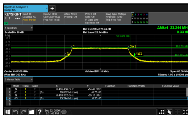
Figure 194 - 802.11ax HE20 SU LPI Maximum 26 dB EBW
