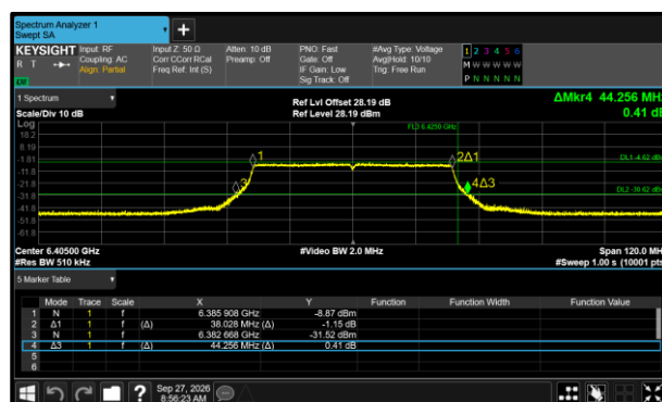
Figure 220 - 802.11ax HE40 SU LPI Maximum 99% OBW
