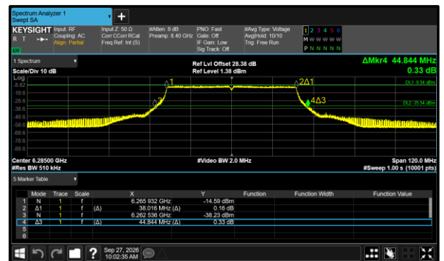
Figure 236 - 802.11ax HE40 SU VLP Maximum 99% OBW
