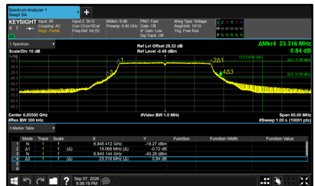
Figure 242 - 802.11ax HE20 SU LPI Maximum 26 dB EBW
