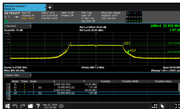
Figure 218 - 802.11ax HE20 SU LPI Maximum 99% OBW
