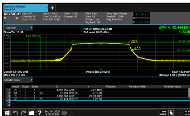
Figure 424 - 802.11ax HE40 SU Minimum 99% OBW
