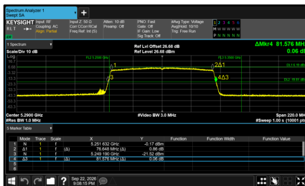
Figure 412 - 802.11ax HE80 SU Minimum 99% OBW
