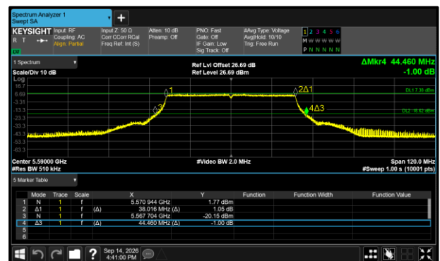
Figure 425 - 802.11ax HE40 SU Maximum 99% OBW
