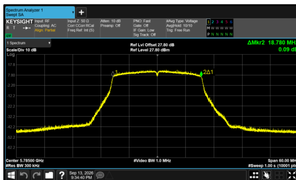
Figure 384 - 802.11ax HE20 SU Minimum 99% OBW
