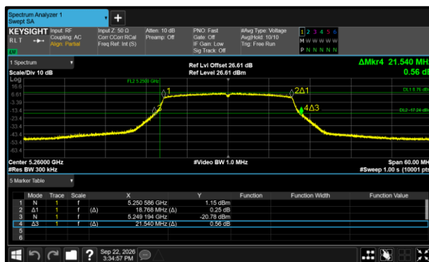
Figure 408 - 802.11ax HE20 SU Minimum 99% OBW
