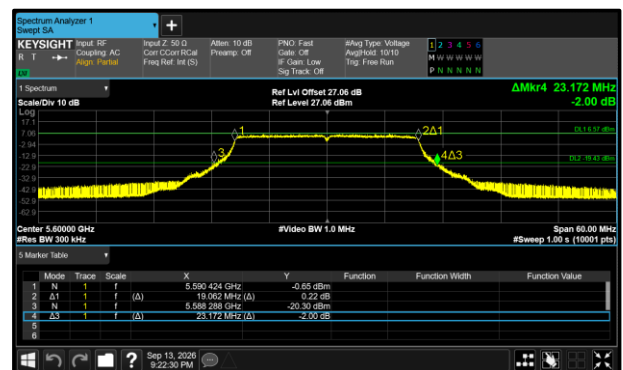
Figure 385 - 802.11ax HE20 SU Maximum 99% OBW
