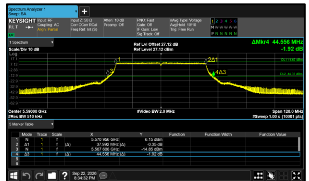
Figure 411 - 802.11ax HE40 SU Maximum 99% OBW
