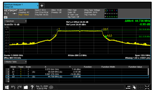
Figure 441 - 802.11ax HE40 SU Maximum 26 dB EBW
