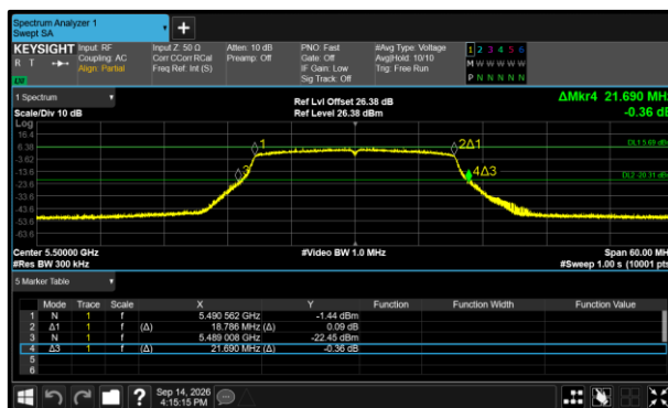
Figure 422 - 802.11ax HE20 SU Minimum 99% OBW
