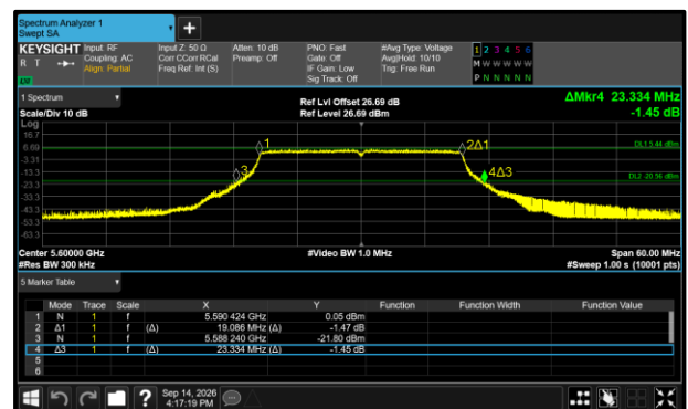
Figure 423 - 802.11ax HE20 SU Maximum 99% OBW
