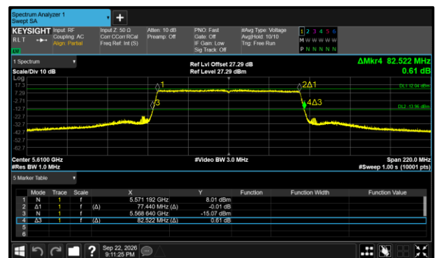
Figure 413 - 802.11ax HE80 SU Maximum 99% OBW
