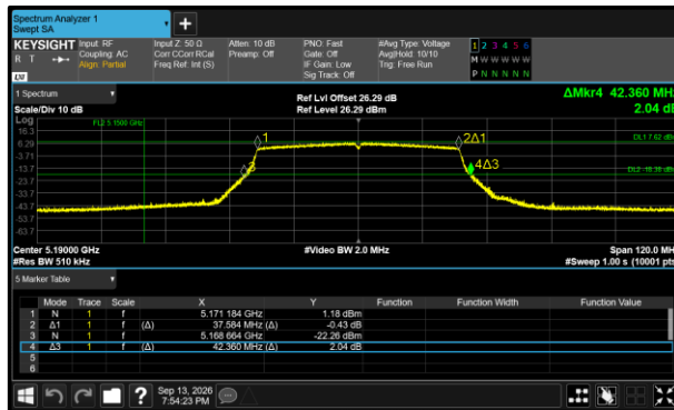
Figure 362 - 802.11ax HE40 SU Minimum 99% OBW
