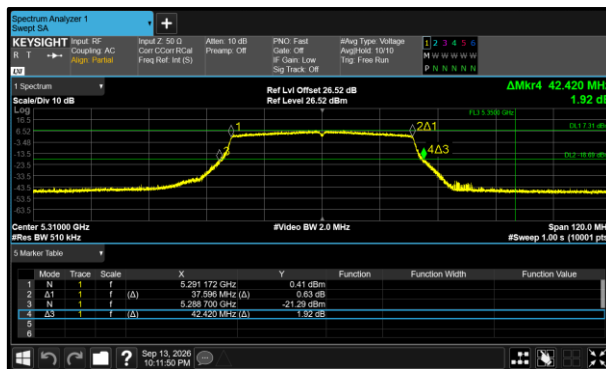
Figure 386 - 802.11ax HE40 SU Minimum 99% OBW
