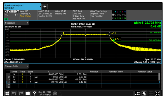
Figure 409 - 802.11ax HE20 SU Maximum 99% OBW
