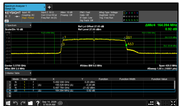
Figure 391 - 802.11ax HE160 SU Maximum 99% OBW
