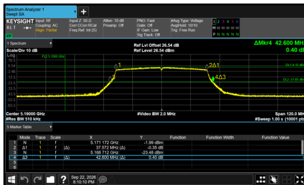
Figure 410 - 802.11ax HE40 SU Minimum 99% OBW
