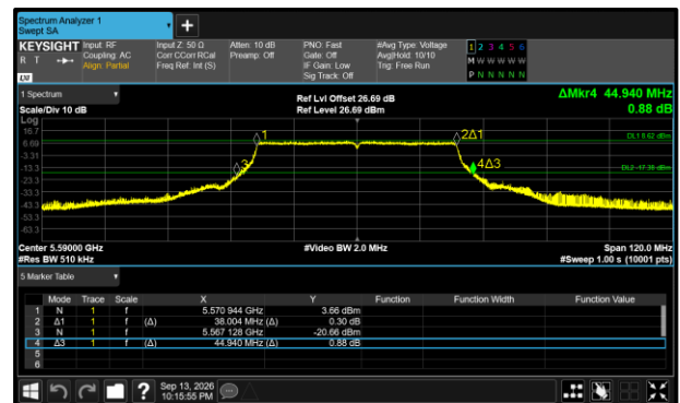
Figure 387 - 802.11ax HE40 SU Maximum 99% OBW
