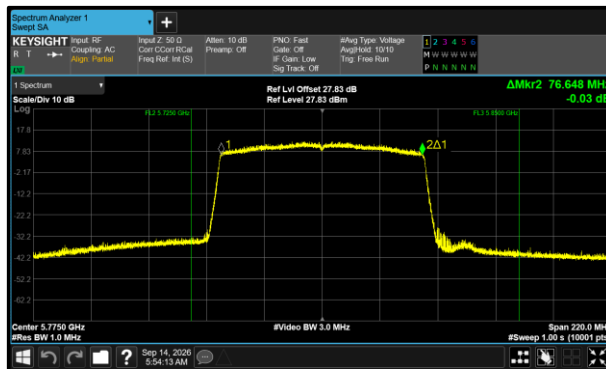
Figure 364 - 802.11ax HE80 SU Minimum 99% OBW
