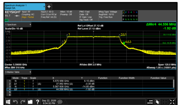
Figure 489 - 802.11ax HE40 SU Maximum 26 dB EBW
