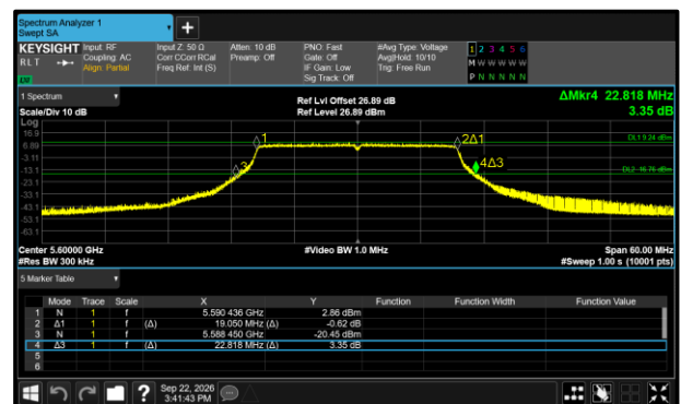
Figure 487 - 802.11ax HE20 SU Maximum 26 dB EBW
