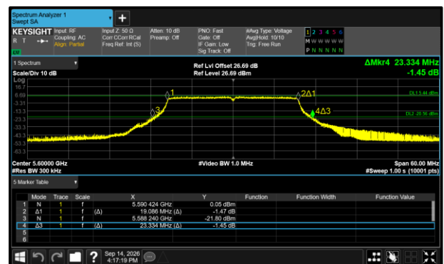
Figure 501 - 802.11ax HE20 SU Maximum 26 dB EBW
