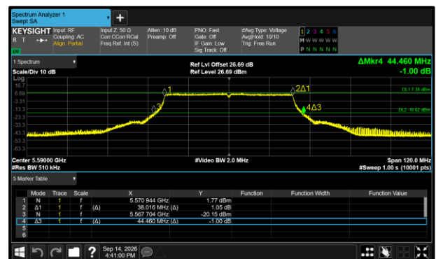
Figure 503 - 802.11ax HE40 SU Maximum 26 dB EBW
