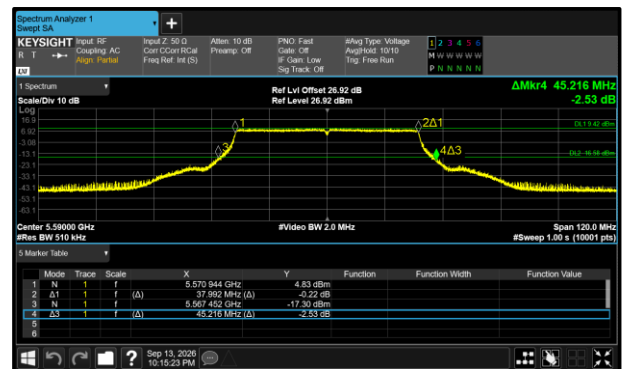
Figure 465 - 802.11ax HE40 SU Maximum 26 dB EBW
