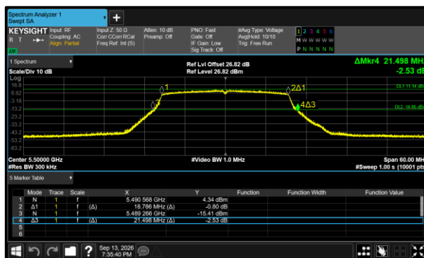
Figure 360 - 802.11ax HE20 SU Minimum 99% OBW
