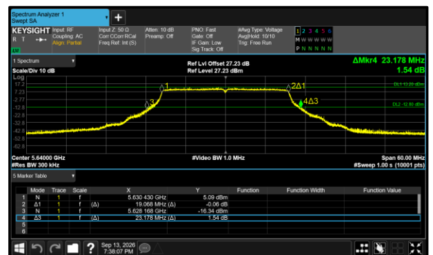
Figure 361 - 802.11ax HE20 SU Maximum 99% OBW
