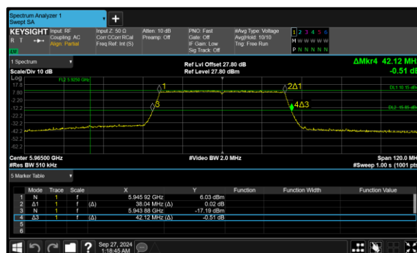
Figure 42 - 802.11ax HE40 SU SP Maximum 99% OBW
