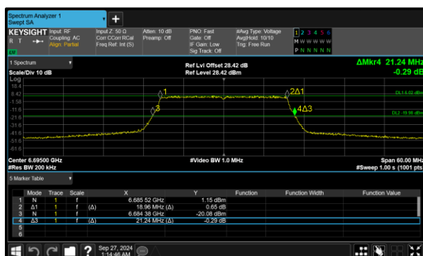
Figure 39 - 802.11ax HE20 SU SP Minimum 99% OBW
