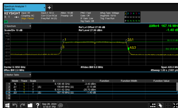
Figure 38 - 802.11ax HE160 SU LPI Maximum 99% OBW
