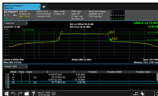
Figure 16 - 802.11ax HE40 SU SP Maximum 26 dB EBW
