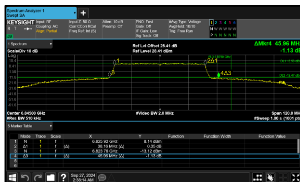
Figure 116 - 802.11ax HE40 SU SP Maximum 26 dB EBW
