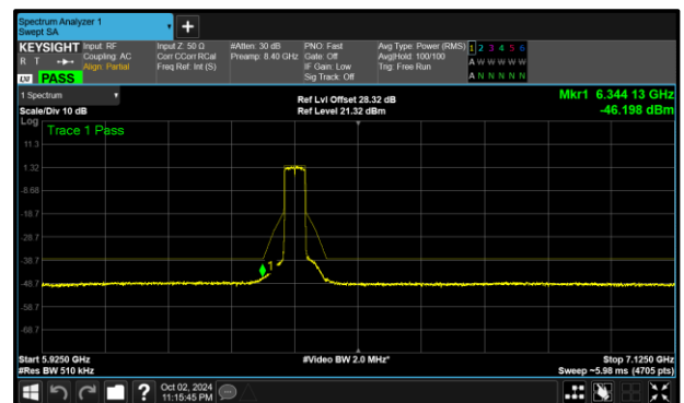
Figure 312 - B (Core 1) 802.11ax HE40 SU SP 6405 MHz (CH91)
