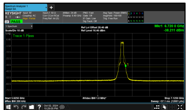
Figure 292 - A (Core 0) 802.11ax HE20 SU SP 6695 MHz (CH149)
