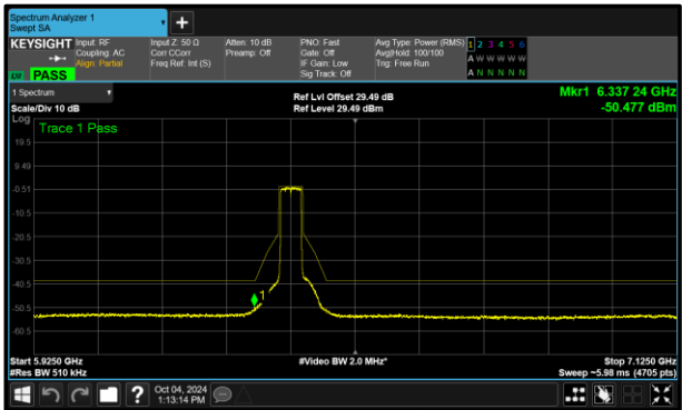
Figure 342 - B (Core 1) 802.11ax HE40 SU SP 6405 MHz (CH91)
