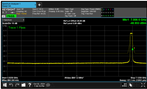
Figure 284 - A (Core 0) 802.11ax HE20 SU LPI 6995 MHz (CH209)
