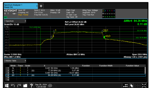
Figure 245 - 802.11ax HE80 SU Maximum 99% OBW
