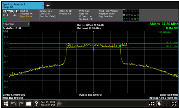
Figure 200 - 802.11ax HE40 SU Minimum 6 dB EBW
