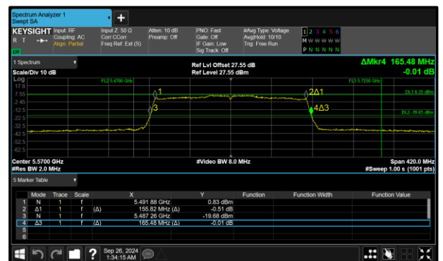
Figure 247 - 802.11ax HE160 SU Maximum 99% OBW
