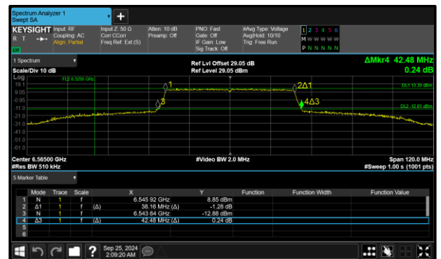
Figure 26 - 802.11ax HE40 SU SP Maximum 26 dB EBW
