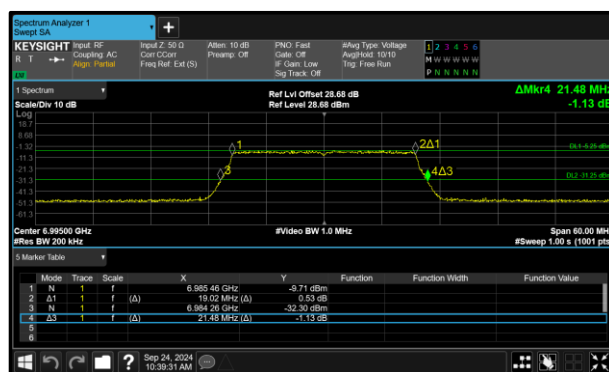
Figure 4 - 802.11ax HE20 SU LPI Maximum 26 dB EBW
