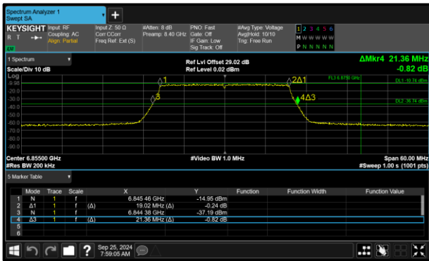
Figure 44 - 802.11ax HE20 SU VLP Maximum 99% OBW
