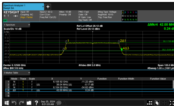
Figure 45 - 802.11ax HE40 SU VLP Minimum 99% OBW
