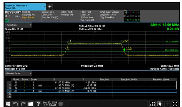
Figure 16 - 802.11ax HE40 SU VLP Maximum 26 dB EBW
