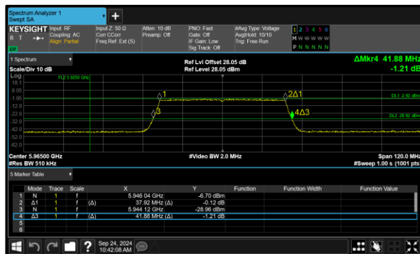
Figure 35 - 802.11ax HE40 SU LPI Minimum 99% OBW
