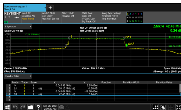
Figure 56 - 802.11ax HE40 SU SP Maximum 99% OBW
