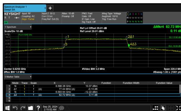
Figure 58 - 802.11ax HE80 SU SP Maximum 99% OBW
