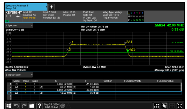
Figure 46 - 802.11ax HE40 SU VLP Maximum 99% OBW
