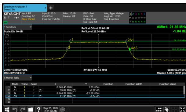
Figure 97 - 802.11ax HE20 SU SP Minimum 99% OBW
