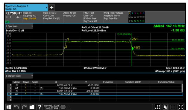
Figure 136 - 802.11ax HE160 SU LPI Maximum 99% OBW
