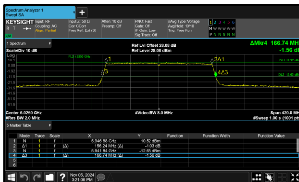
Figure 103 - 802.11ax HE160 SU SP Minimum 99% OBW
