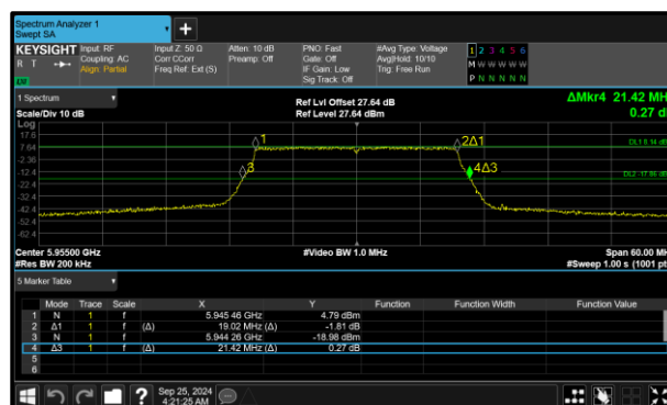
Figure 122 - 802.11ax HE20 SU SP Maximum 26 dB EBW
