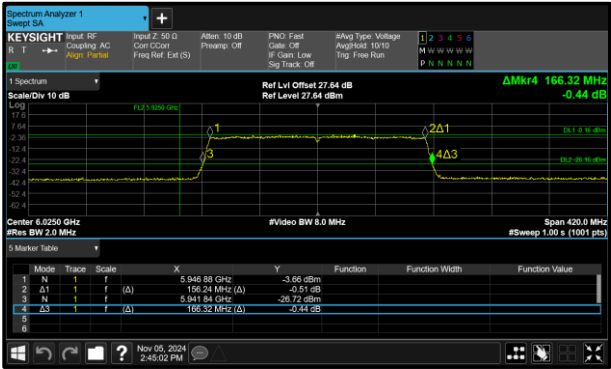
Figure 89 - 802.11ax HE160 SU LPI Minimum 99% OBW
