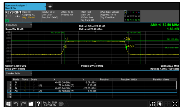
Figure 134 - 802.11ax HE80 SU LPI Maximum 99% OBW
