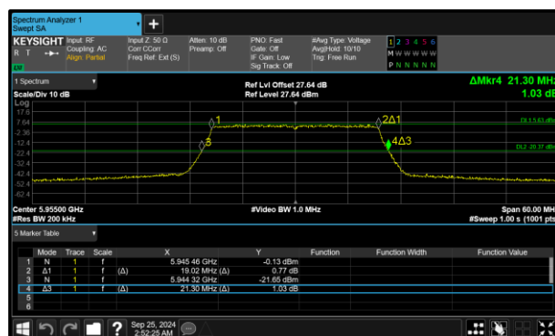
Figure 98 - 802.11ax HE20 SU SP Maximum 99% OBW
