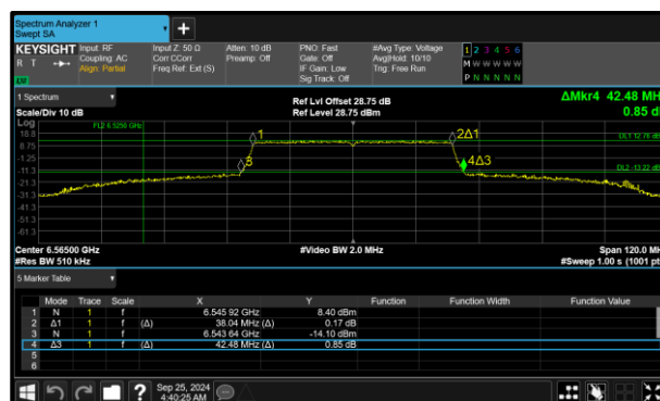
Figure 124 - 802.11ax HE40 SU SP Maximum 26 dB EBW
