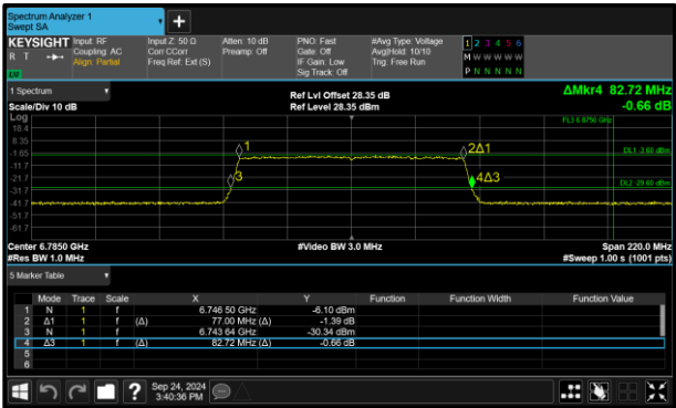
Figure 87 - 802.11ax HE80 SU LPI Minimum 99% OBW
