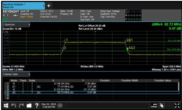
Figure 88 - 802.11ax HE80 SU LPI Maximum 99% OBW
