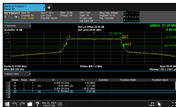
Figure 146 - 802.11ax HE20 SU SP Maximum 99% OBW
