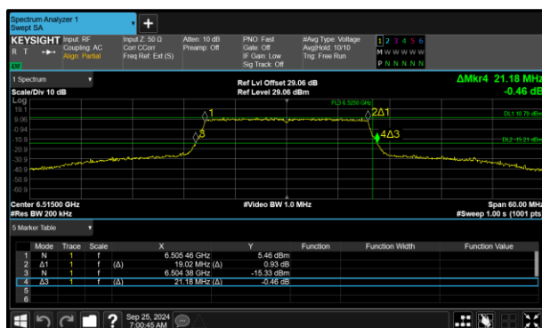
Figure 121 - 802.11ax HE20 SU SP Minimum 26 dB EBW
