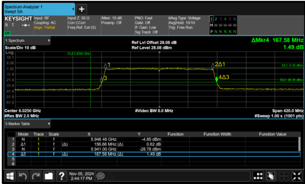
Figure 90 - 802.11ax HE160 SU LPI Maximum 99% OBW
