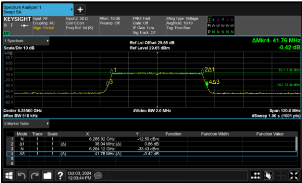
Figure 153 - 802.11ax HE40 SU LPI Minimum 26 dB EBW
