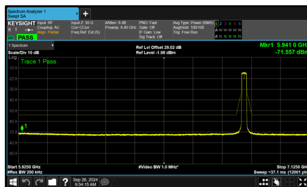
Figure 283 - A (Core 0) 802.11ax HE20 SU LPI 6855 MHz (CH181)
