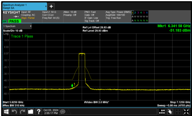
Figure 340 - A (Core 0) 802.11ax HE40 SU SP 6405 MHz (CH91)
