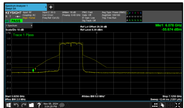
Figure 322 - A (Core 0) 802.11ax HE160 SU LPI 6345 MHz (CH79)
