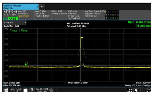
Figure 299 - A (Core 0) 802.11ax HE20 SU VLP 6535 MHz (CH117)
