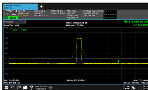
Figure 304 - B (Core 1) 802.11ax HE40 SU LPI 6525 MHz (CH115)
