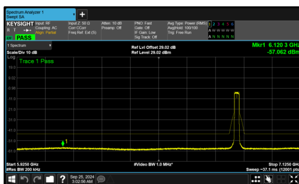
Figure 309 - A (Core 0) 802.11ax HE20 SU SP 6855 MHz (CH181)
