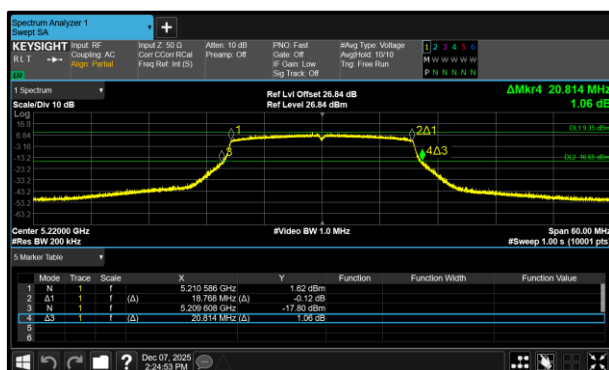
Figure 334 - 802.11ax HE20 SU Minimum 26 dB EBW
