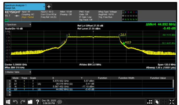
Figure 353 - 802.11ax HE40 SU Maximum 26 dB EBW
