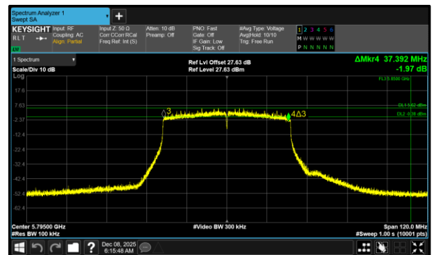
Figure 409 - 802.11ax HE40 SU Maximum 6 dB EBW
