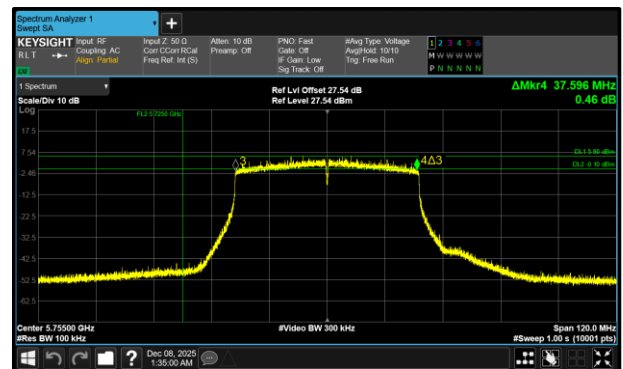
Figure 391 - 802.11ax HE40 SU Maximum 6 dB EBW
