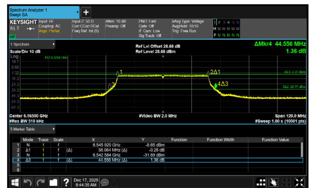
Figure 188 - 802.11ax HE40 SU VLP Maximum 99% OBW
