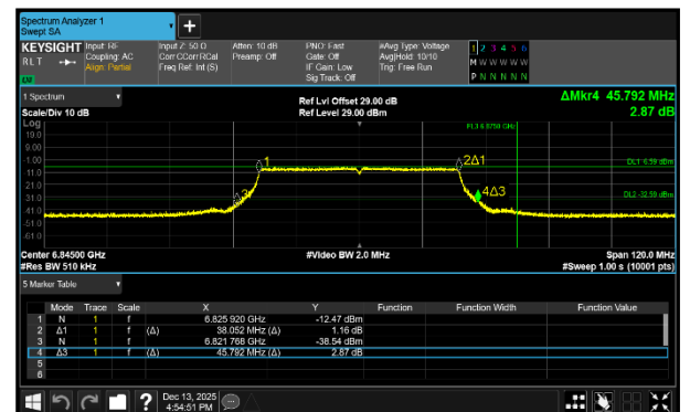
Figure 204 - 802.11ax HE40 SU LPI Maximum 26 dB EBW
