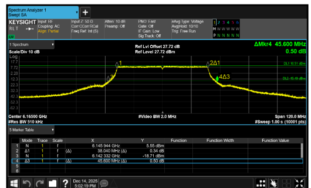
Figure 220 - 802.11ax HE40 SU SP Maximum 26 dB EBW
