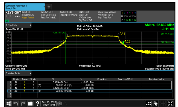
Figure 202 - 802.11ax HE20 SU LPI Maximum 26 dB EBW
