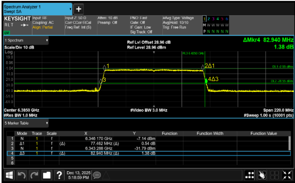
Figure 206 - 802.11ax HE80 SU LPI Maximum 26 dB EBW
