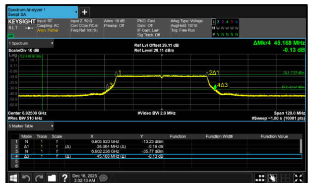
Figure 236 - 802.11ax HE40 SU VLP Maximum 26 dB EBW
